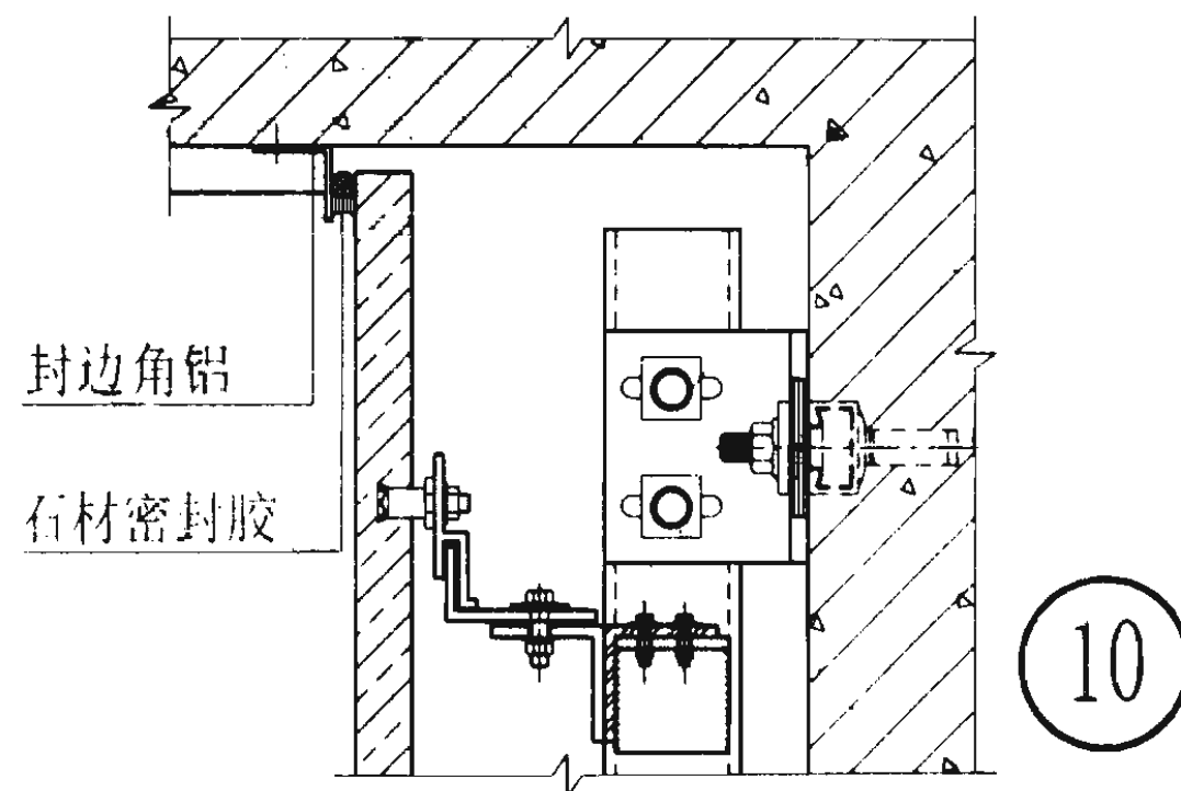
上封顶节点图
