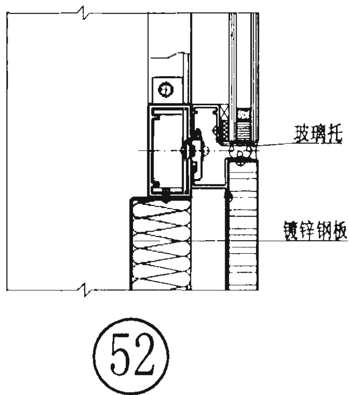
蜂窝结构与玻璃连接节点图
