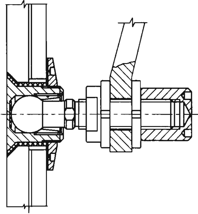
TCXX/XX装配图
