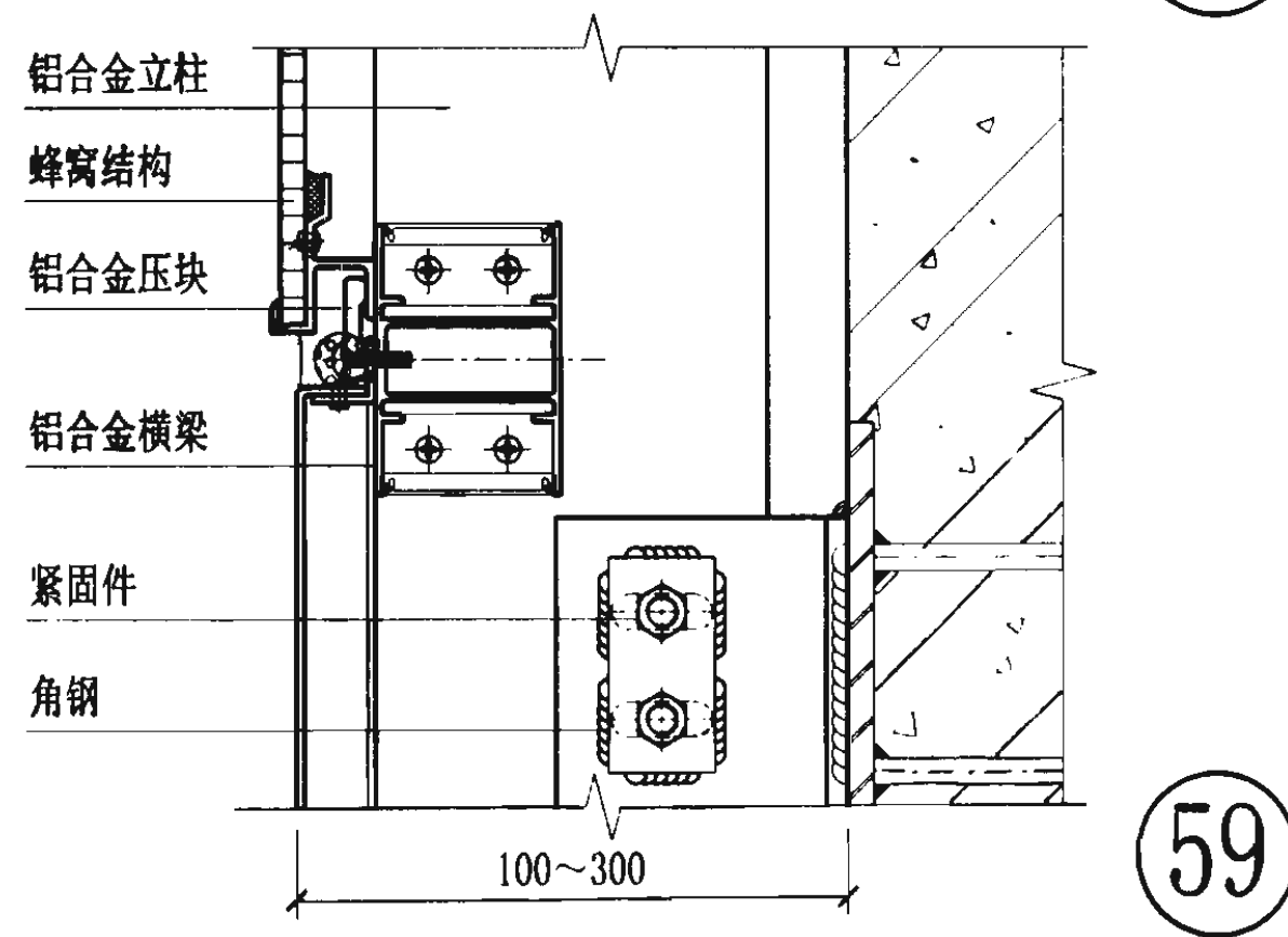
铝合金单板与蜂窝结构连接节点图
