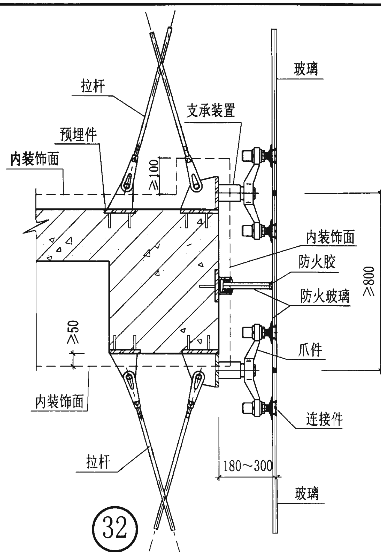
层间梁节点图
