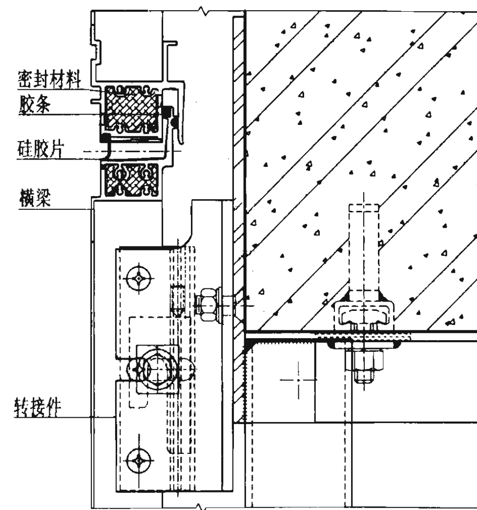
主体结构连接节点图
