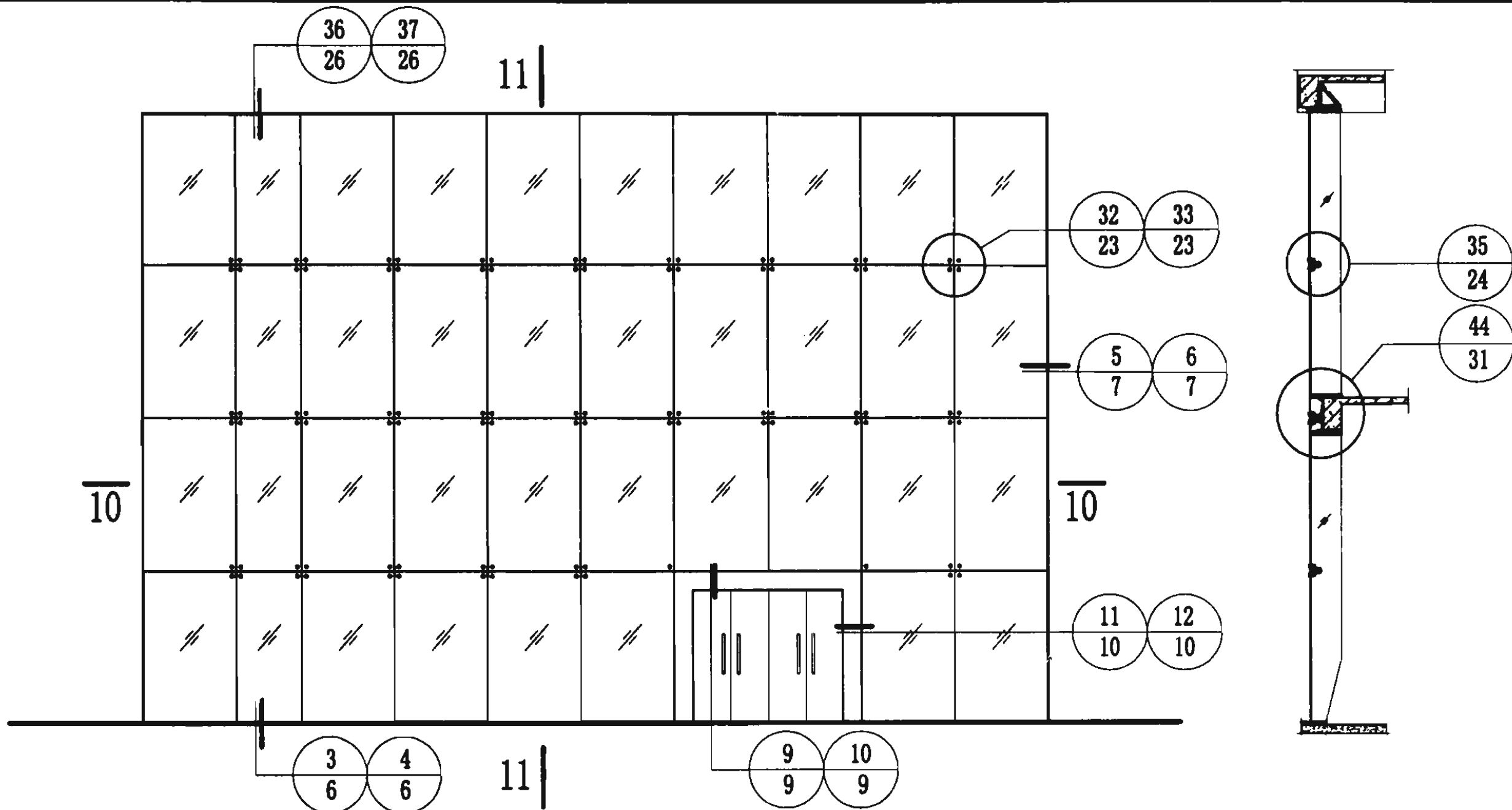
立面示意图
