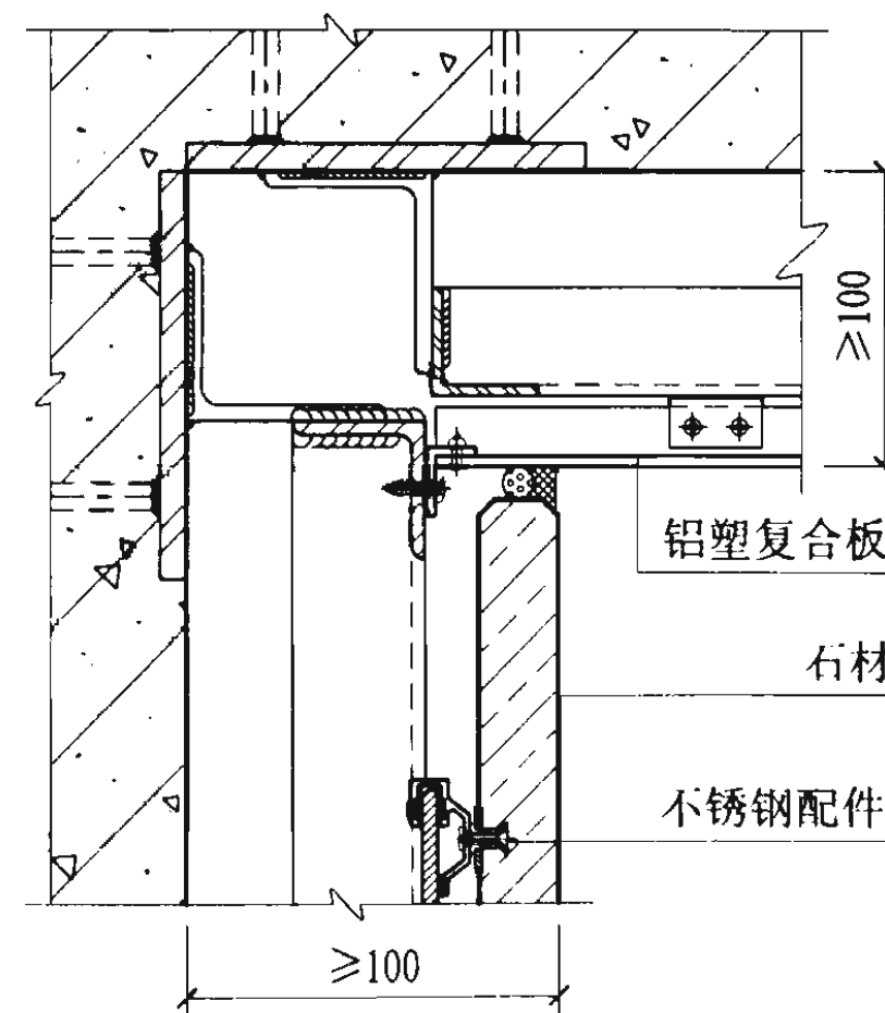
铝塑复合板与石材连接节点图
