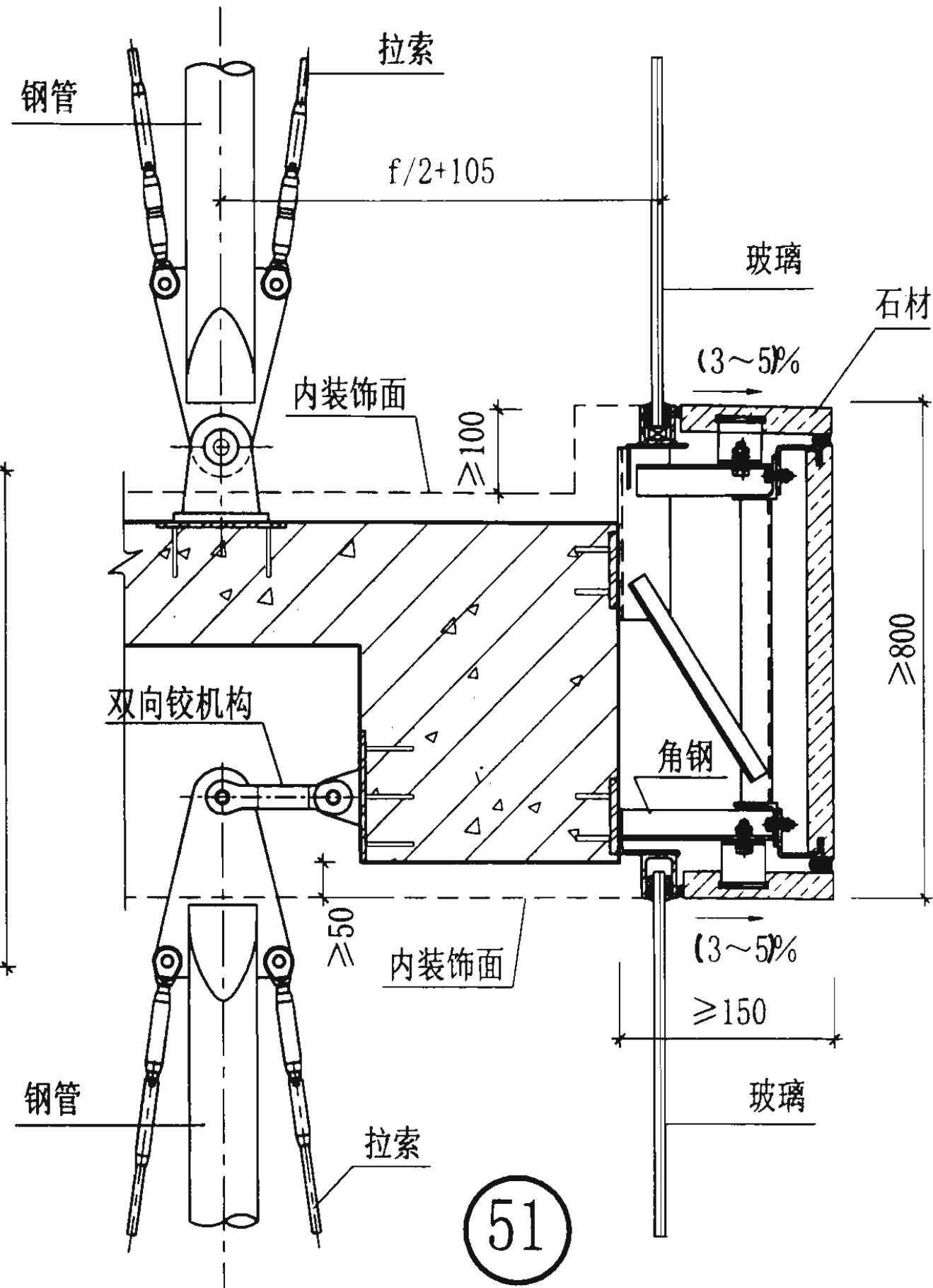
层间梁节点图
