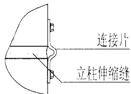
A向局部 防雷装置连接示意图
