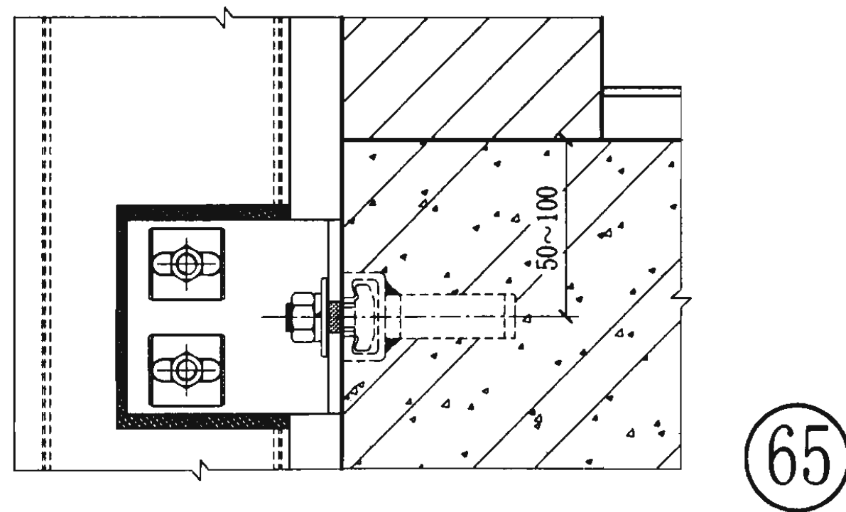
主体结构连接节点图
