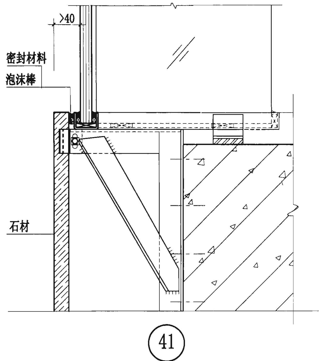
层间梁节点图
