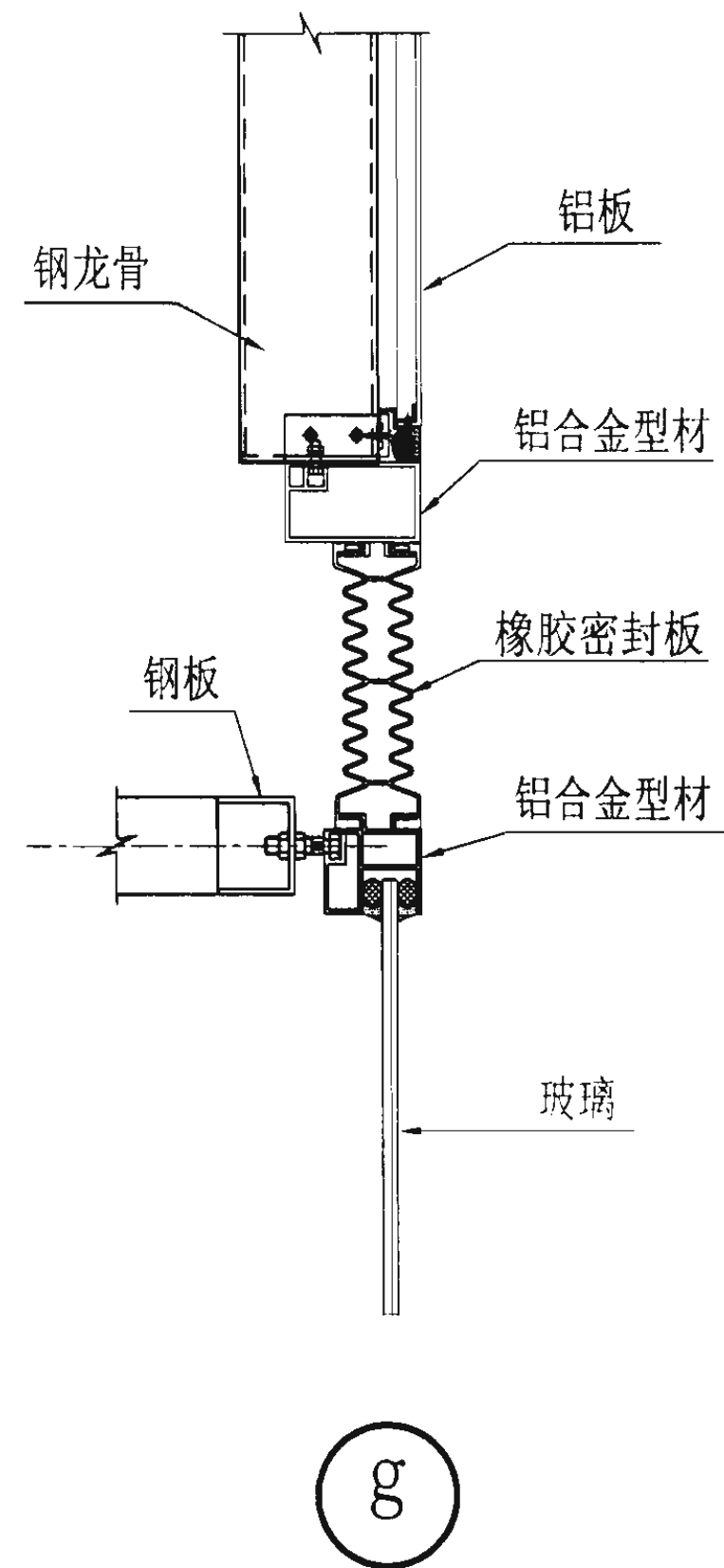
上封顶节点图
