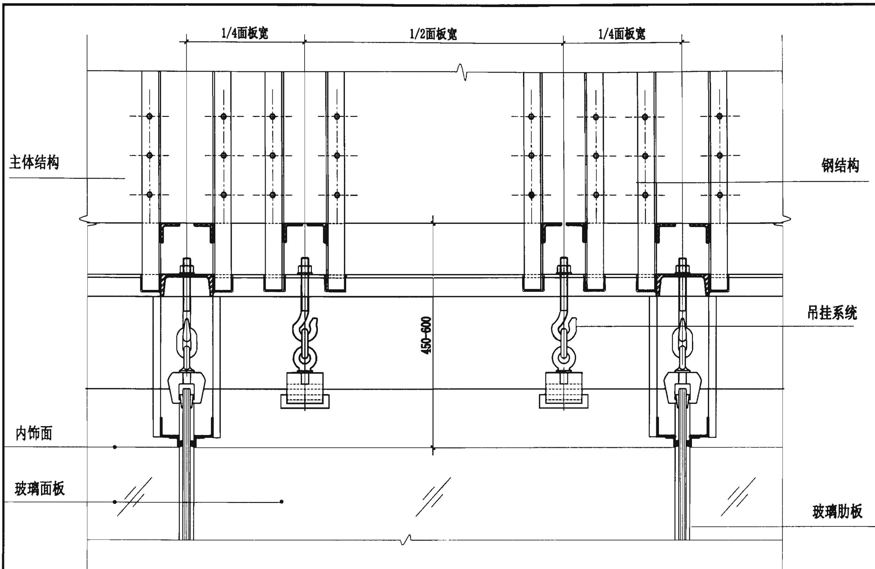
吊具定位图
