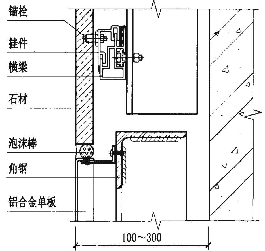
铝合金单板与石材连接节点图
