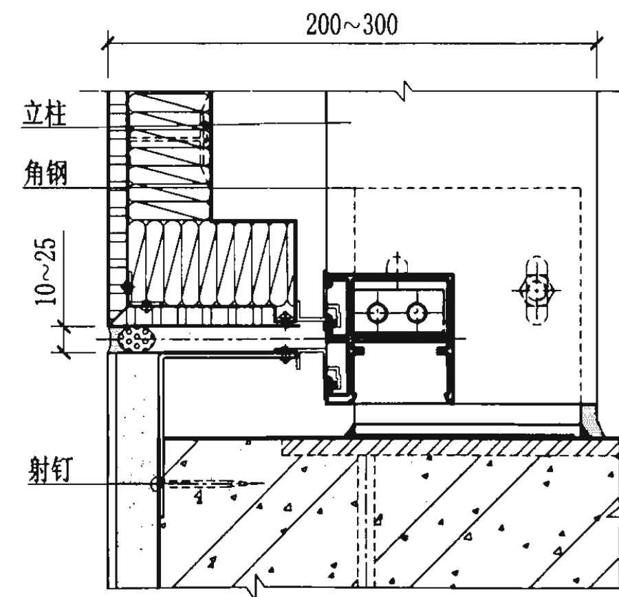
下封底节点图
