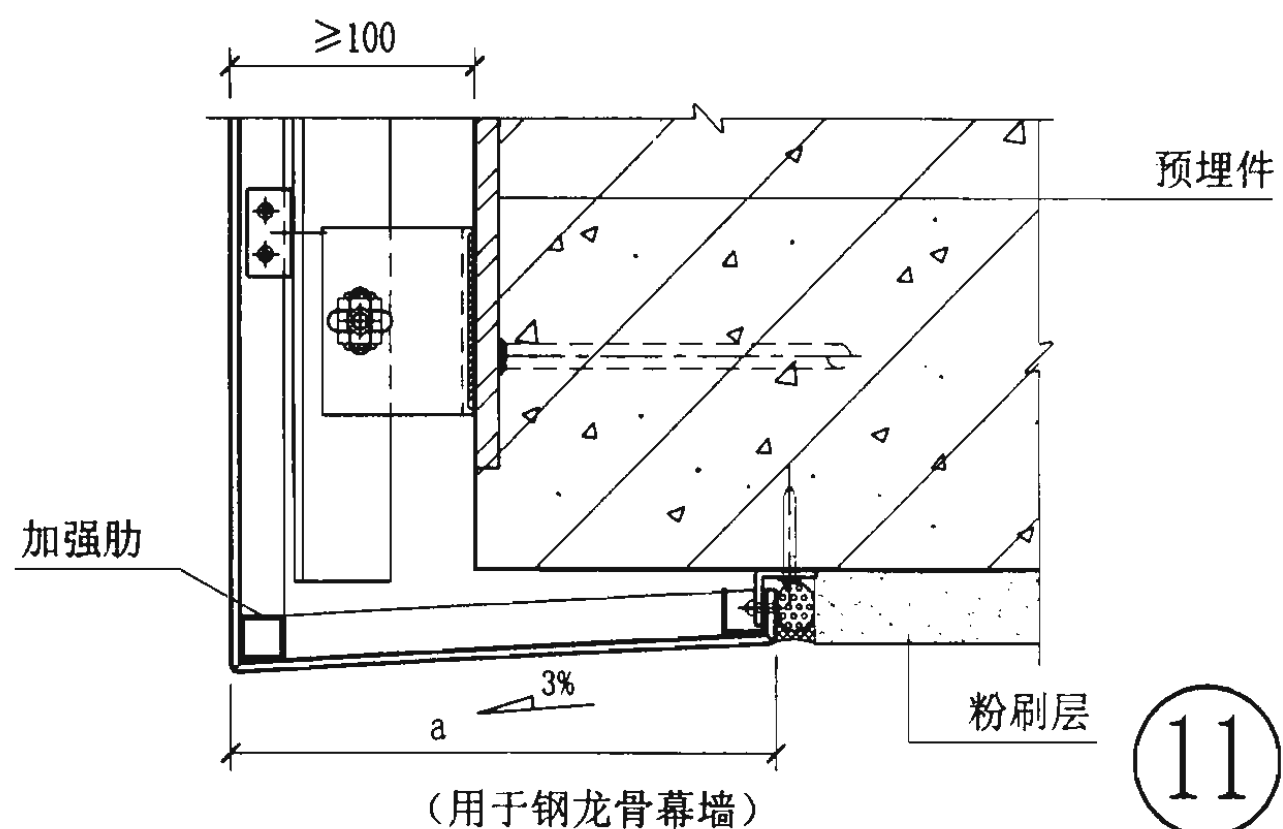
下封底节点图
