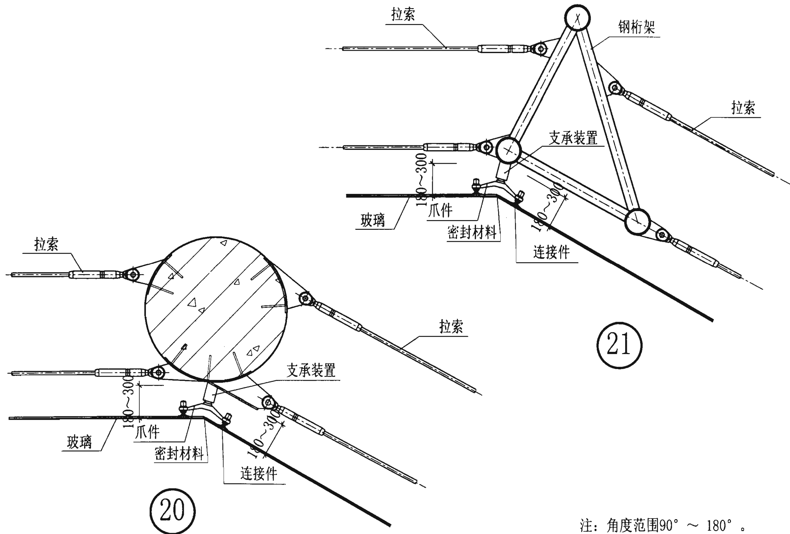
转角部位节点图
