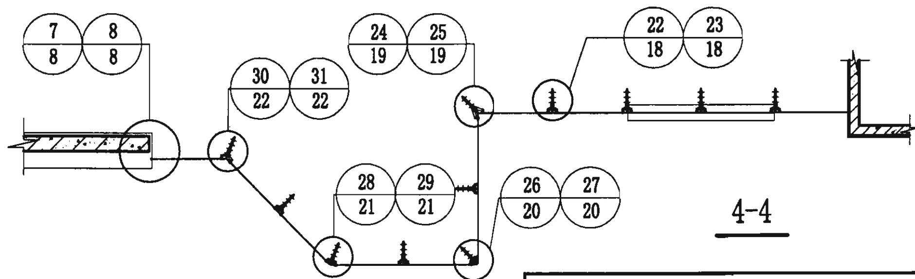
吊挂点支式玻璃幕墙索引图
