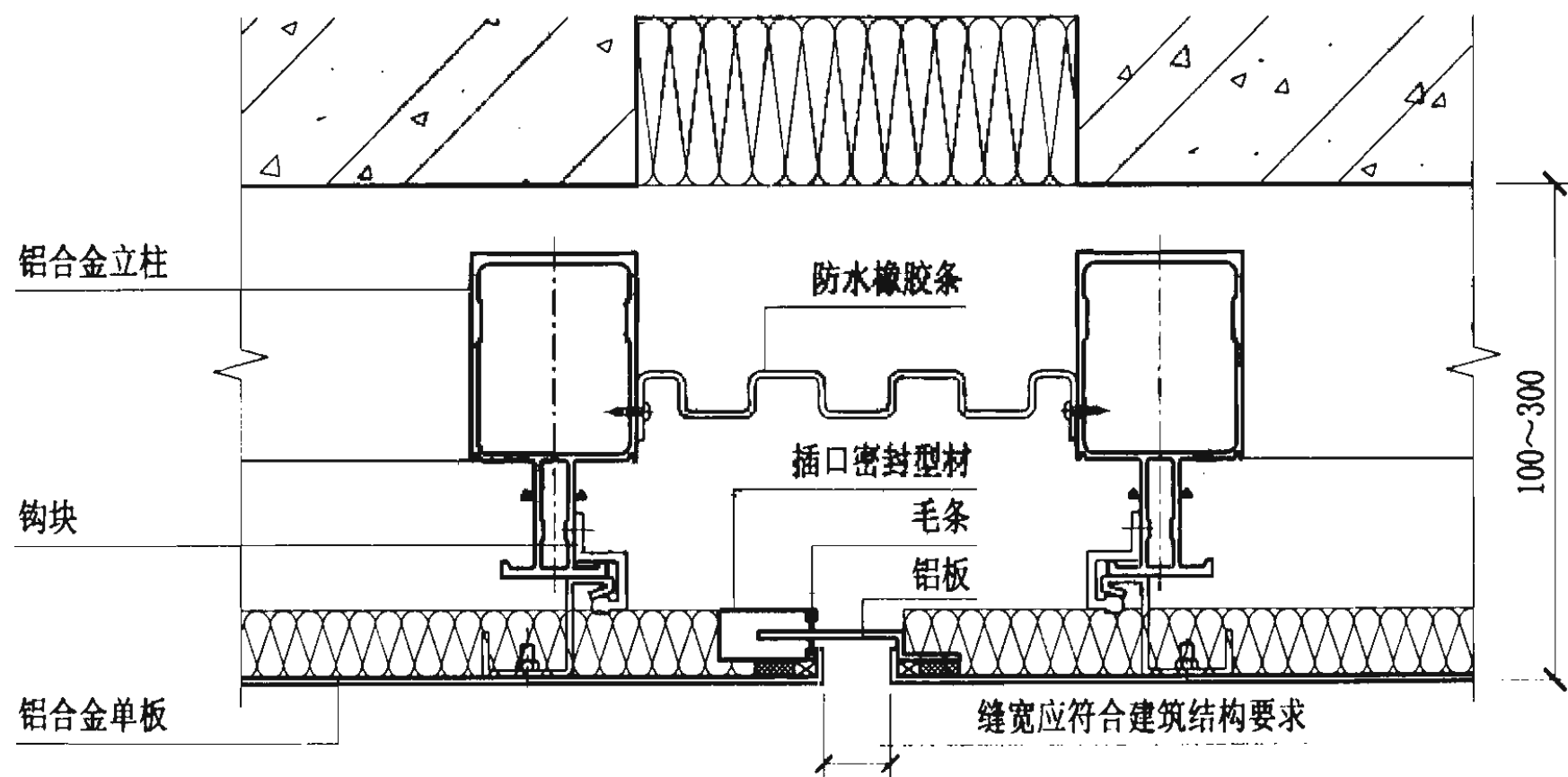
伸缩缝节点图
