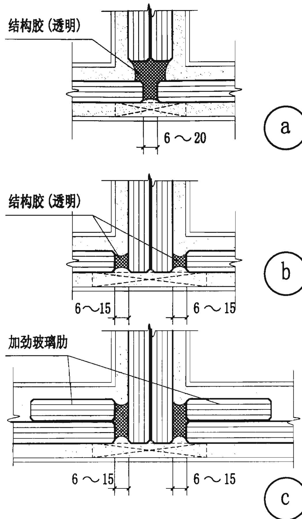
玻璃装配节点图
