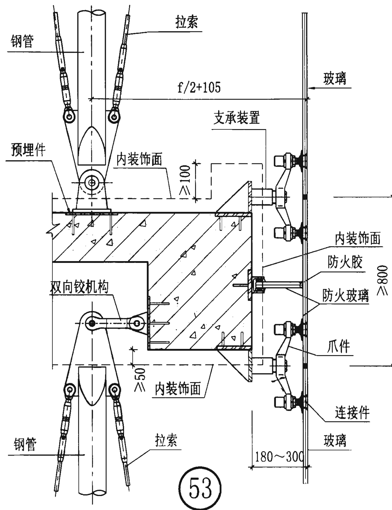
层间梁节点图
