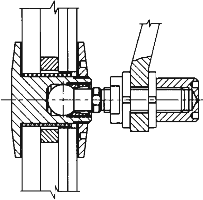
TTXX/XX装配图
