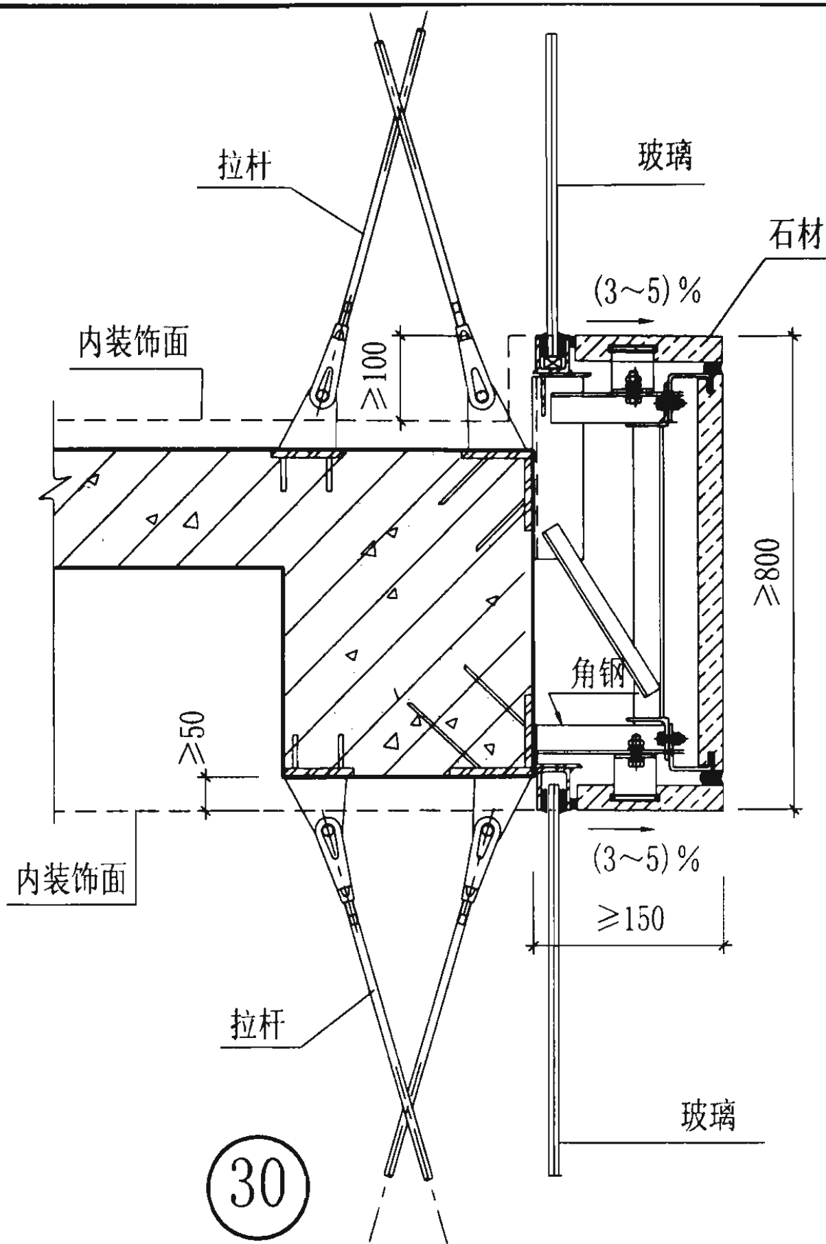
层间梁节点图
