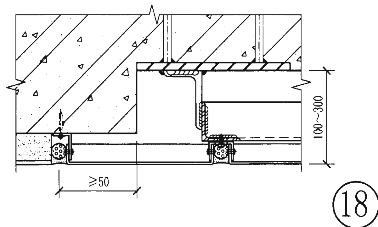
侧封边节点图
