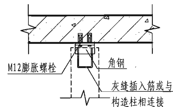
16 砌体墙与板底连接处 需要设置锚固件
