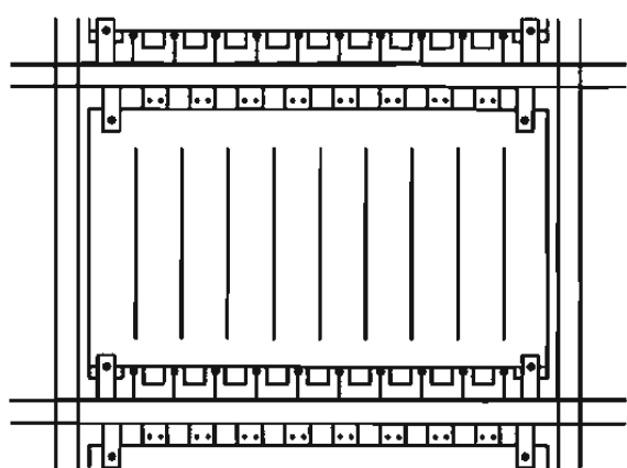
带竖缝的混凝土剪力墙板
