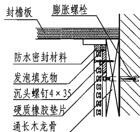
3 檐口
