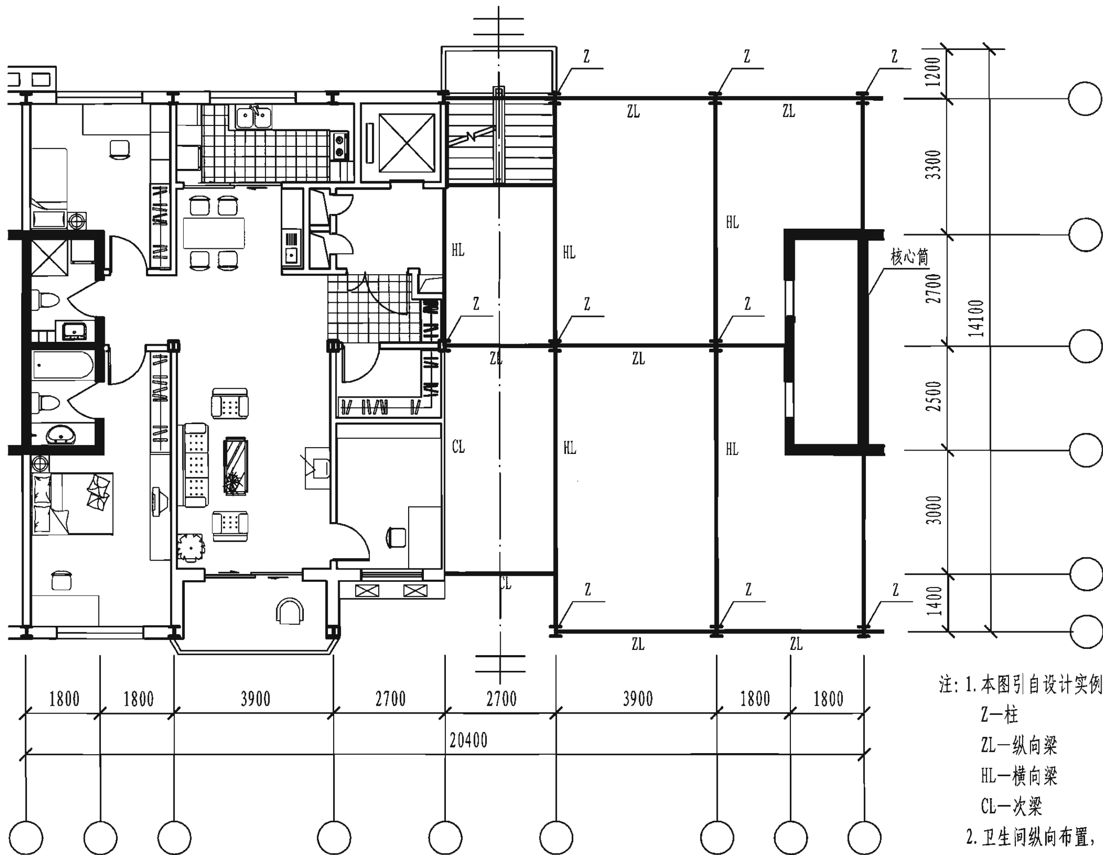
建筑平面图
