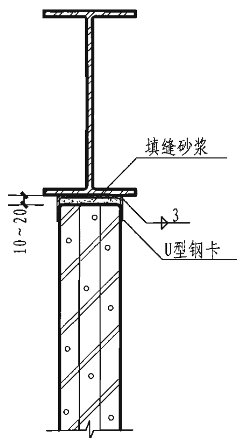
1 隔墙与钢梁对中连接
