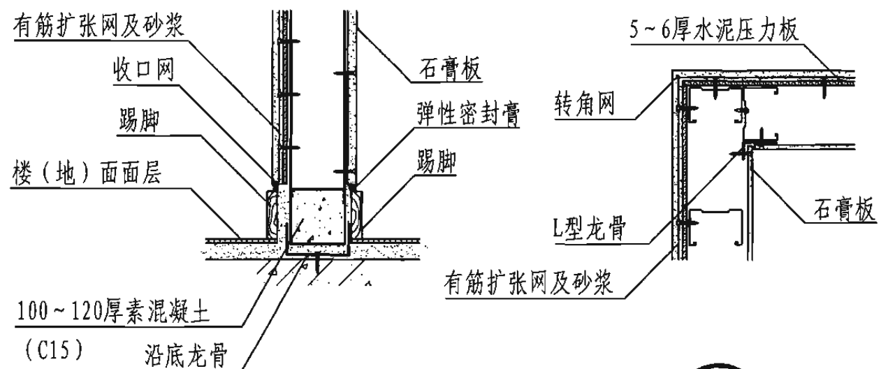
5) 内墙转角
