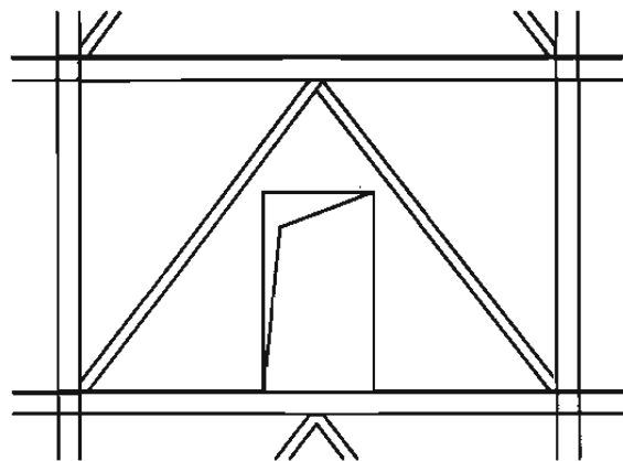
人字中心支撑 (层高较大时)
