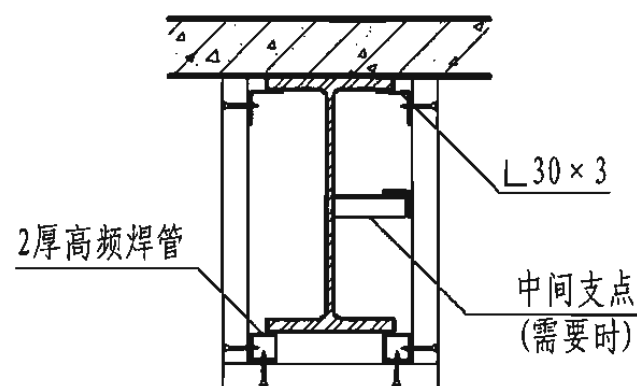
5 防火板包梁
