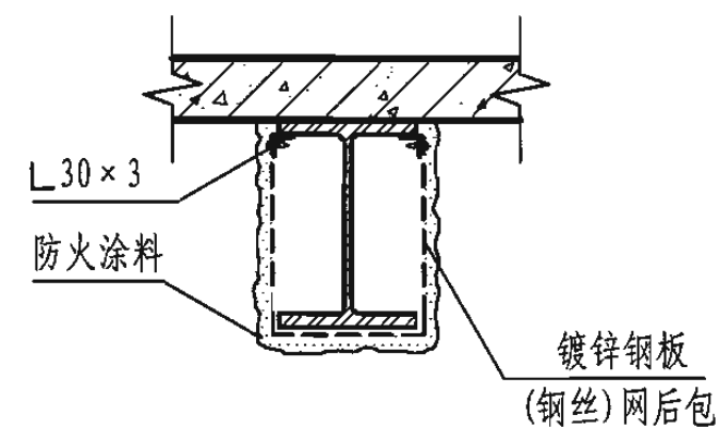
4 板下梁挂网喷涂
