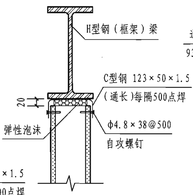
7 墙板与钢梁连接
