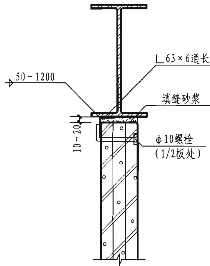
2 隔墙与钢梁对中连接
