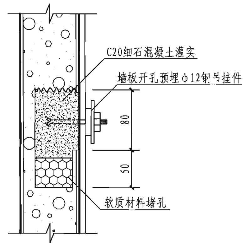
3 墙板预埋钢吊挂件
