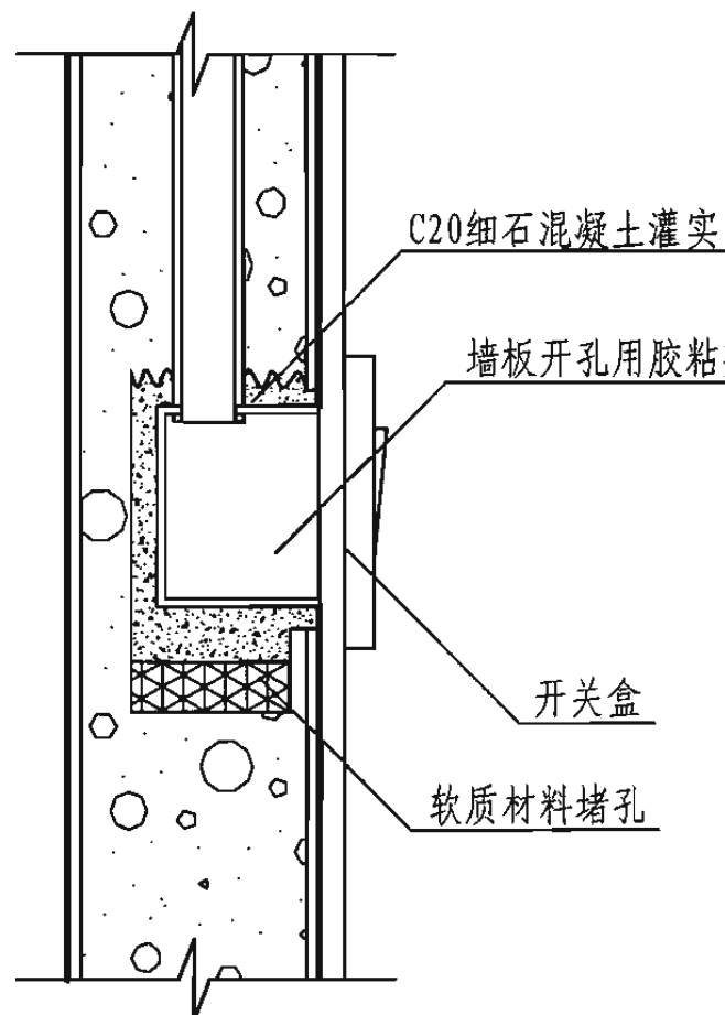
暗线开关敷线安装
