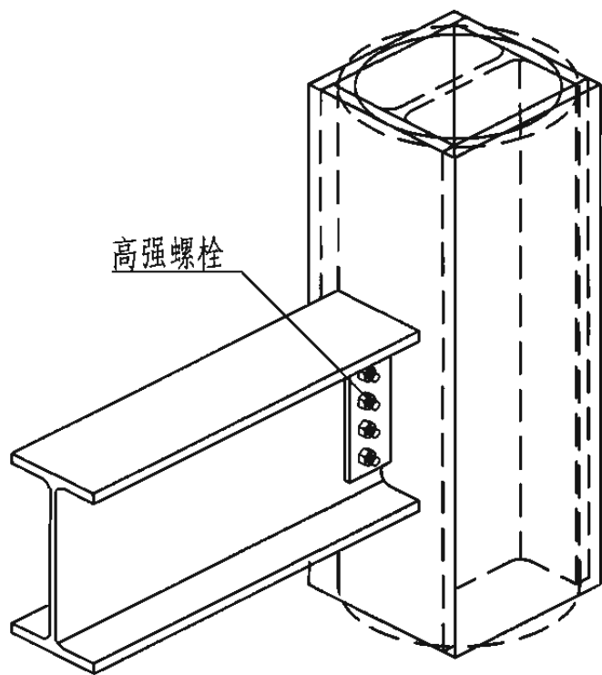
任意截面柱与梁铰接
