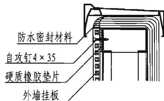
2 女儿墙
