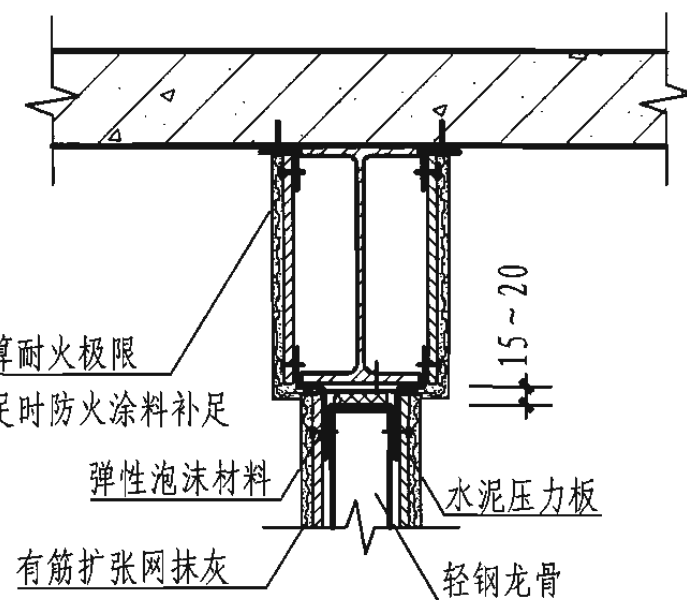
11 轻钢有筋网隔墙对中布置 (可一侧按本做法, 一侧 钉石膏板或其它板)
