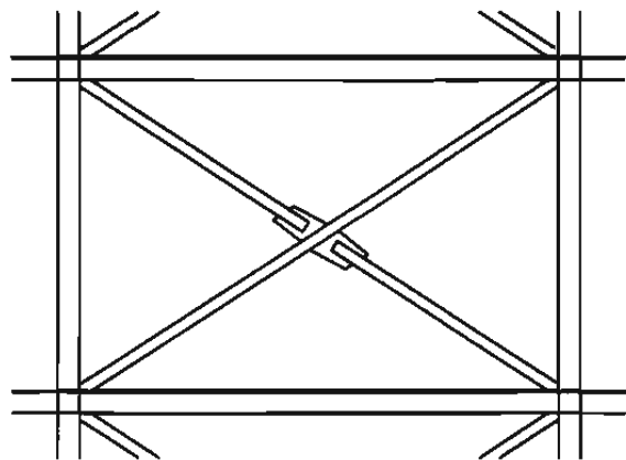
十字交叉中心支撑
