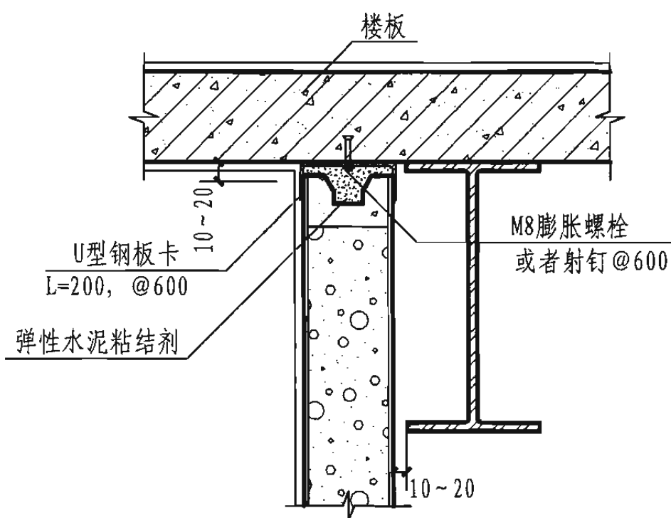
4 隔墙偏置时的连接
