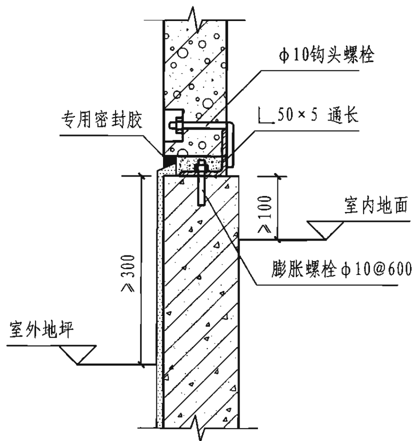
1 外墙竖板墙基部位
