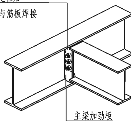
主梁与次梁简支连接
