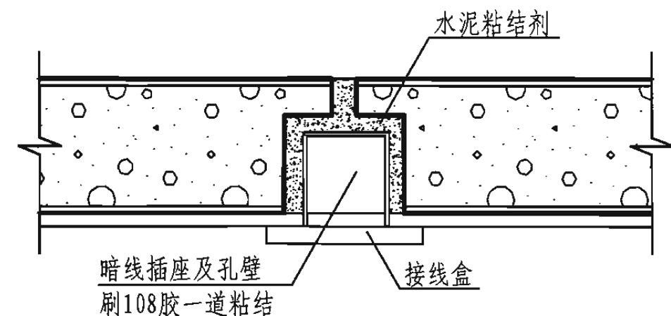
4 板缝安装暗线插座
