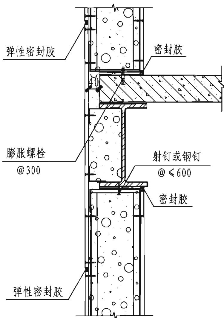
1 外墙楼层处
