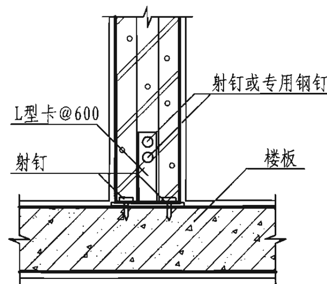
6 隔墙与楼板的连接
