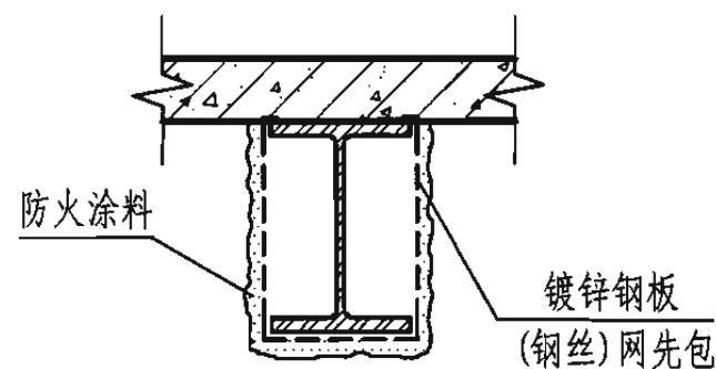
3 板下梁挂网喷涂
