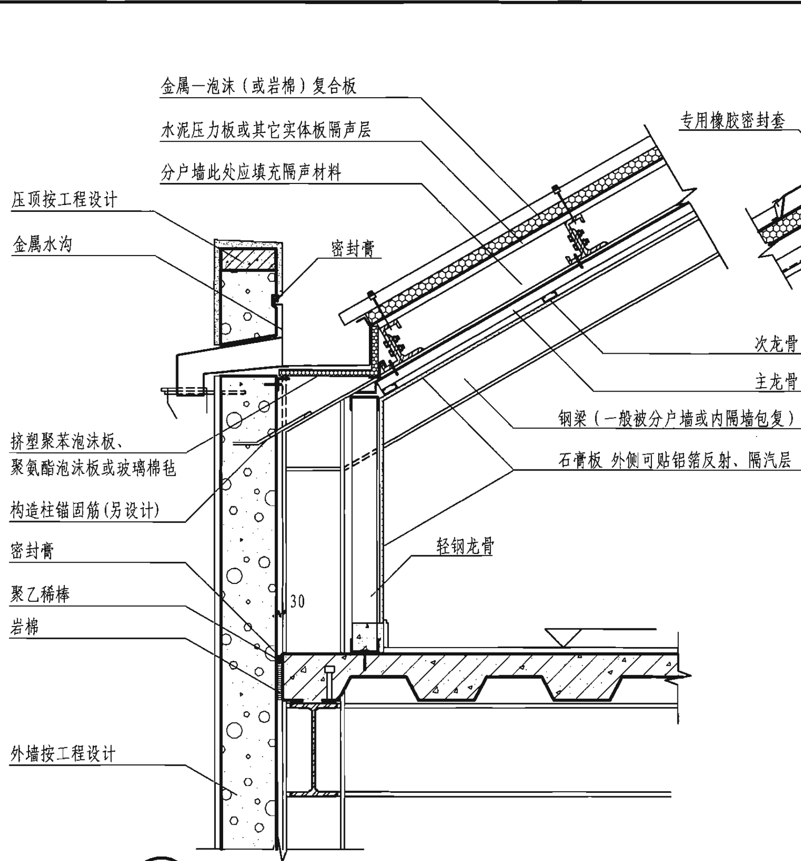
1 利用内部空间的坡屋顶——夹芯板屋面
