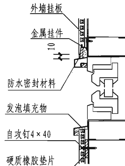
11 窗口
