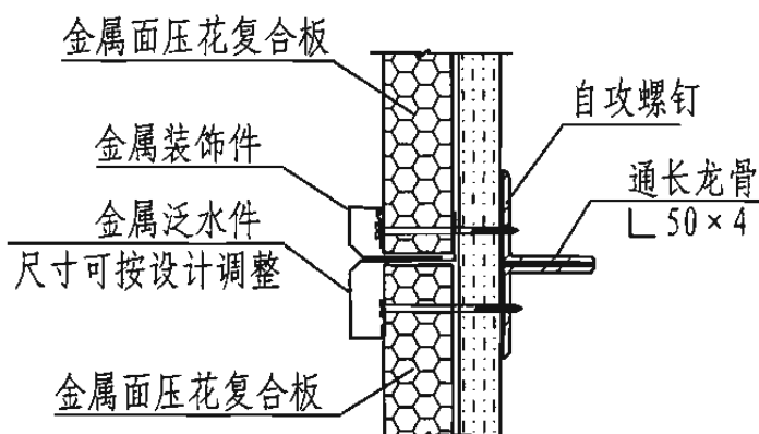
水平接缝装饰线
