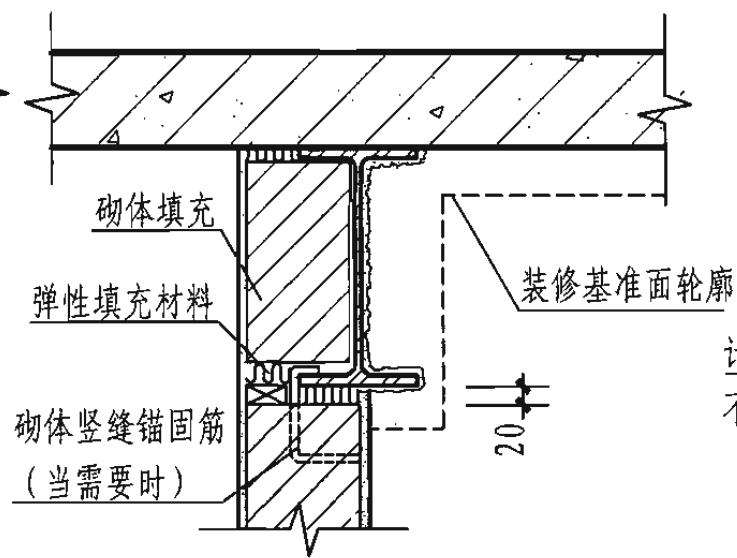
10 砌体墙 偏置
