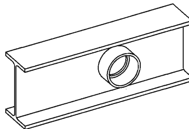
梁腹板上开圆孔后补强
