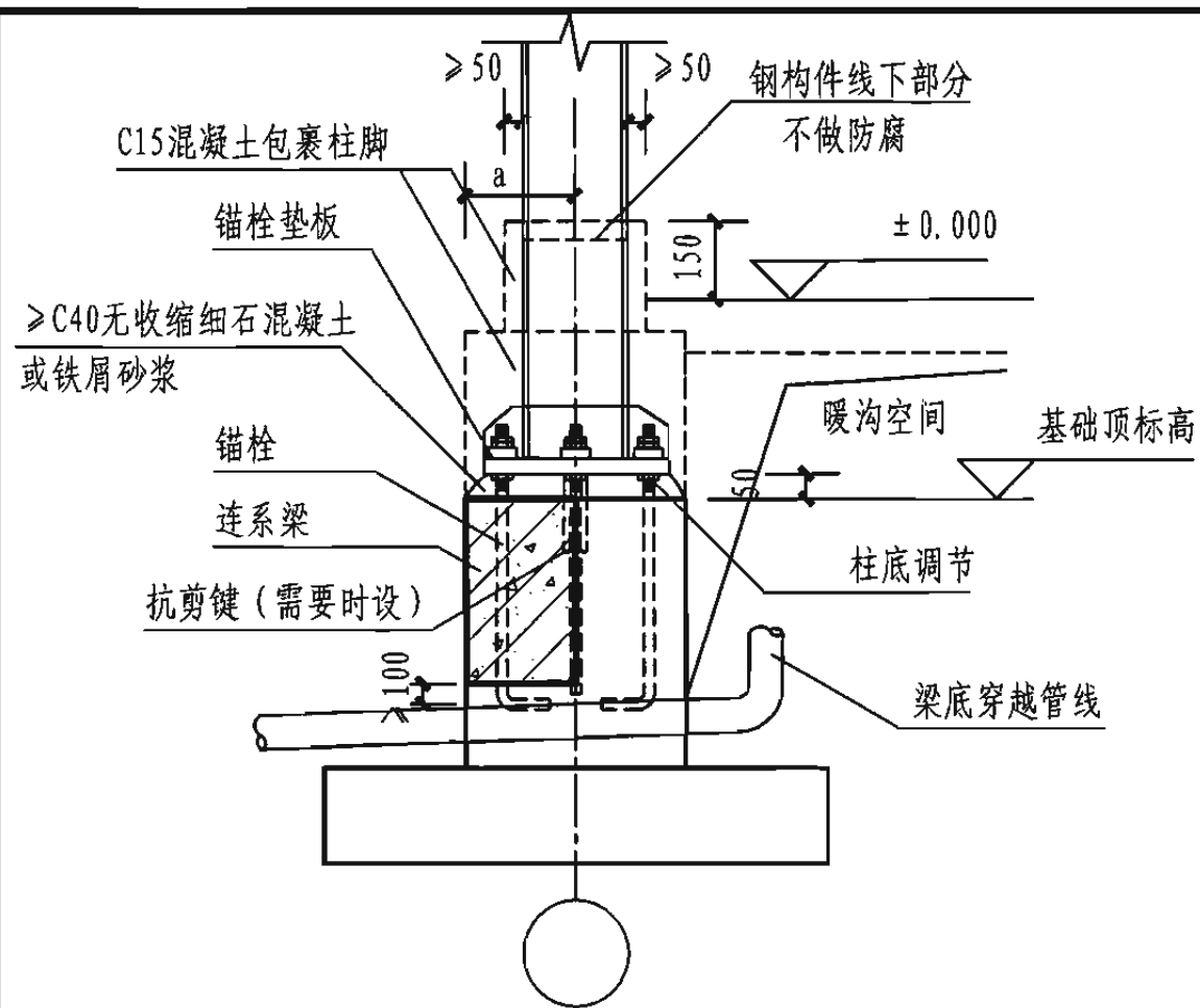
独立基础加连系梁 (适用多层)
