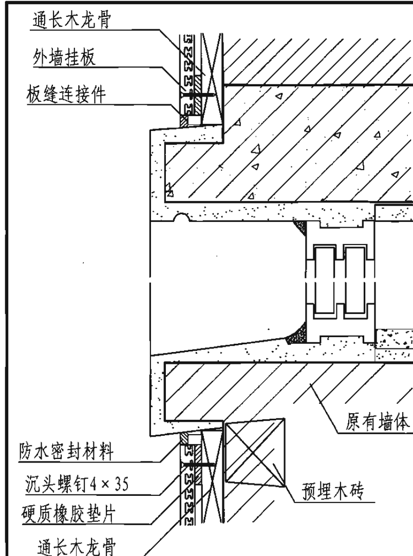
1 窗洞口
