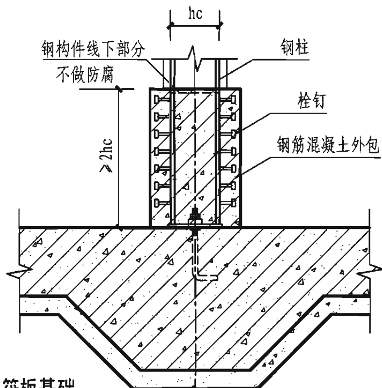
筏板基础 外包式刚性柱脚 (适用多层、中高层)
