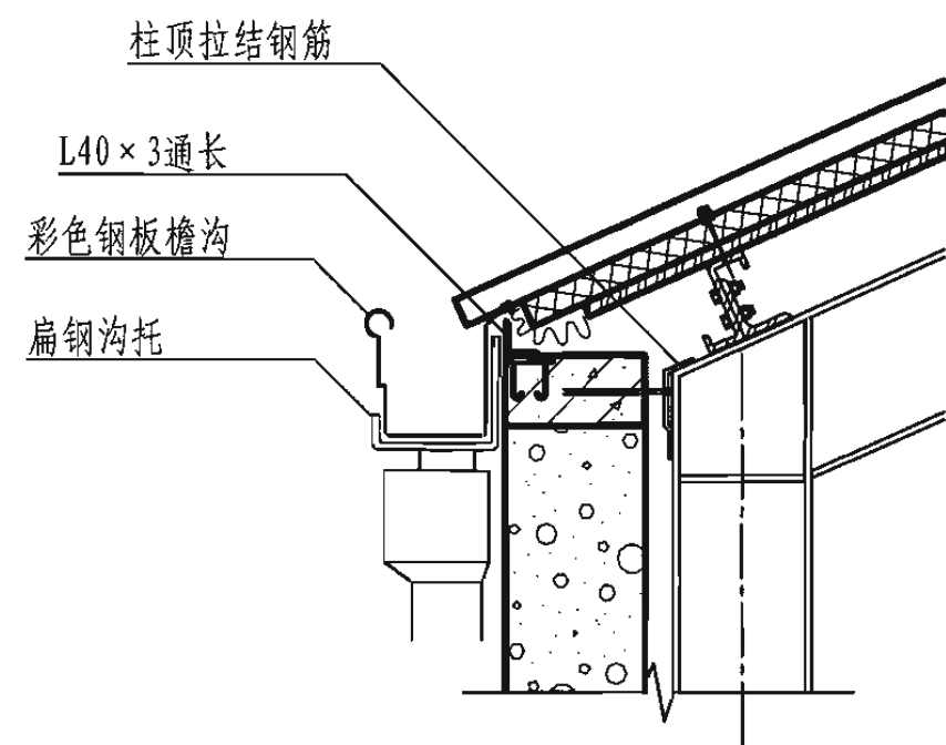
1 金属复合板屋顶外排水檐口
