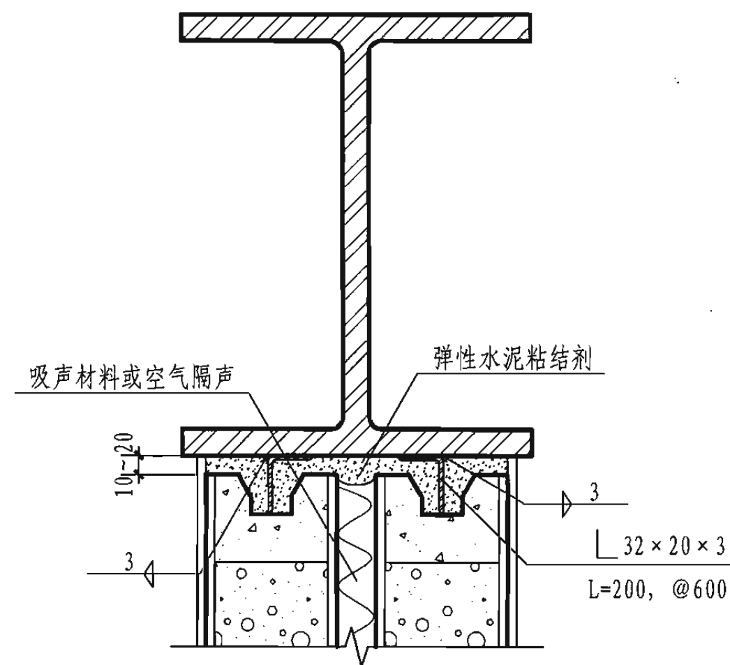
3 分户墙与钢梁连接
