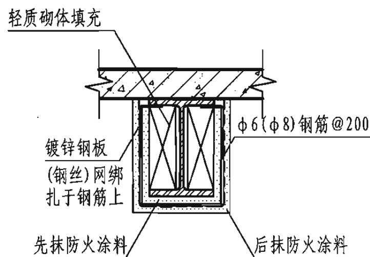
6 成形式防火涂料
