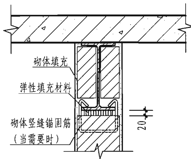
9 砌体墙 对中布置
