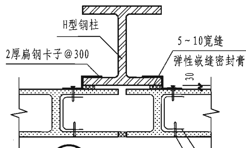
1 墙板与钢柱连接
