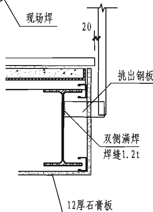
3 梁式楼梯栏杆立柱侧装方法
