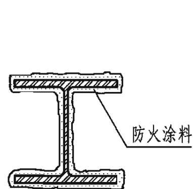
8 防火涂料包柱
