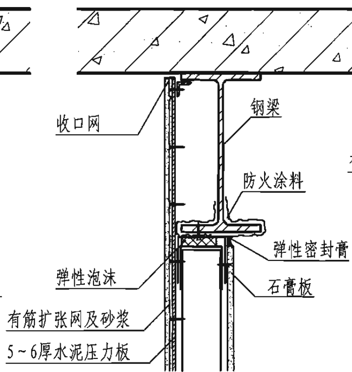
2 轻钢龙骨墙偏置
