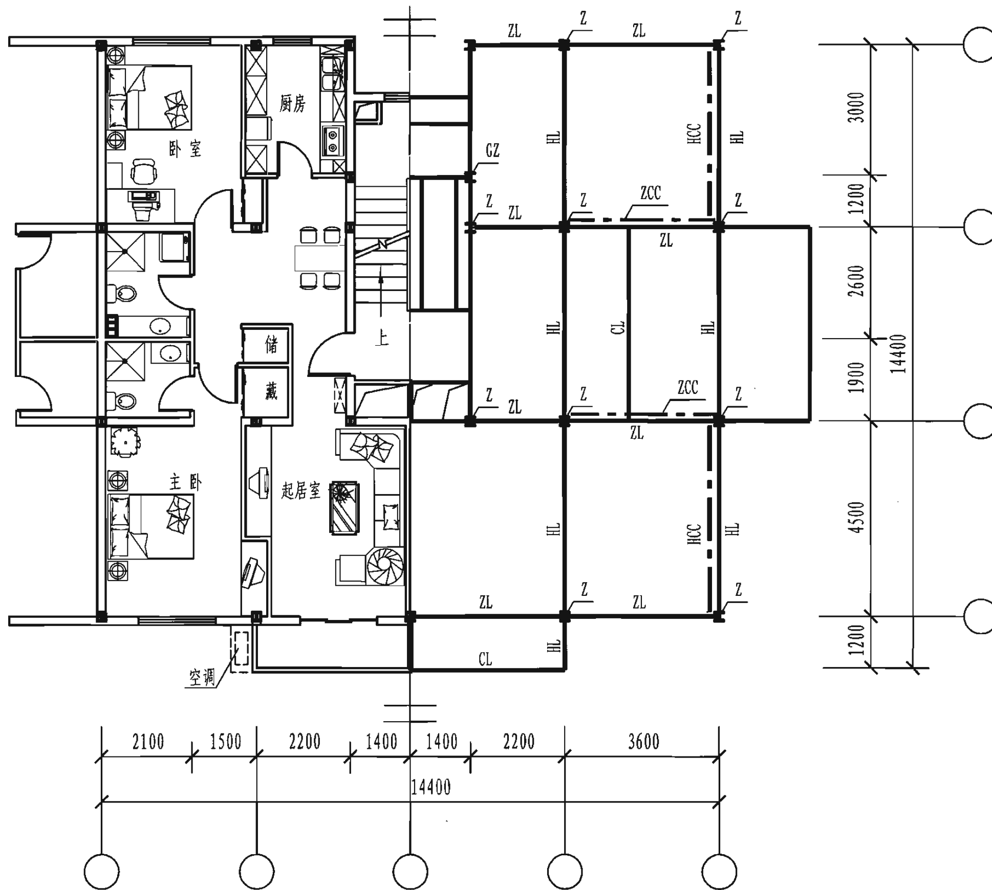
建筑平面图
