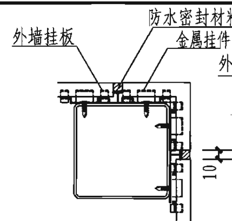
4 阳角
