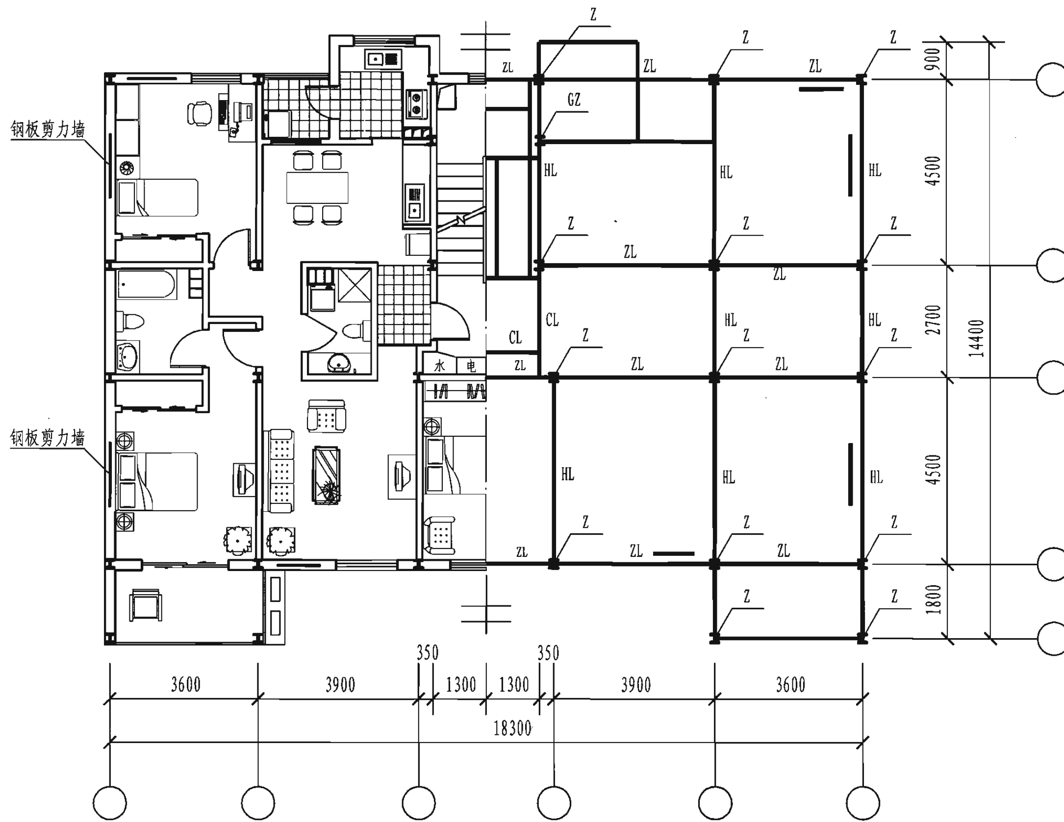
建筑平面图
