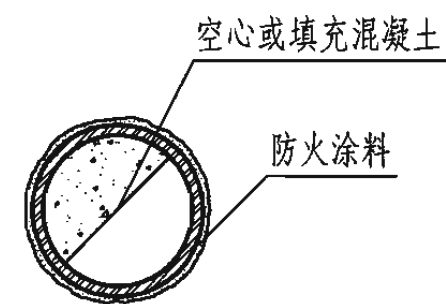
11 防火涂料包柱
