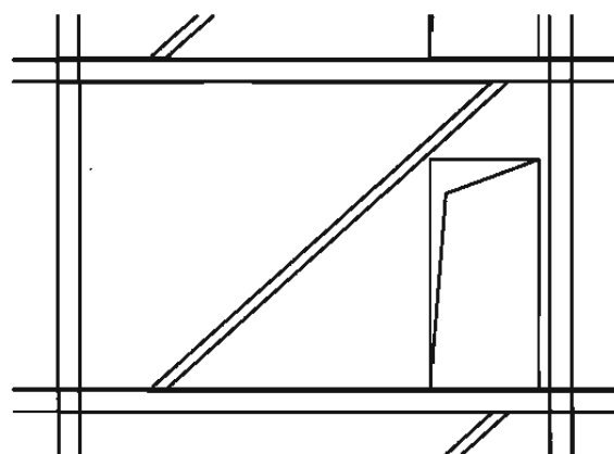
单斜杆偏心支撑
