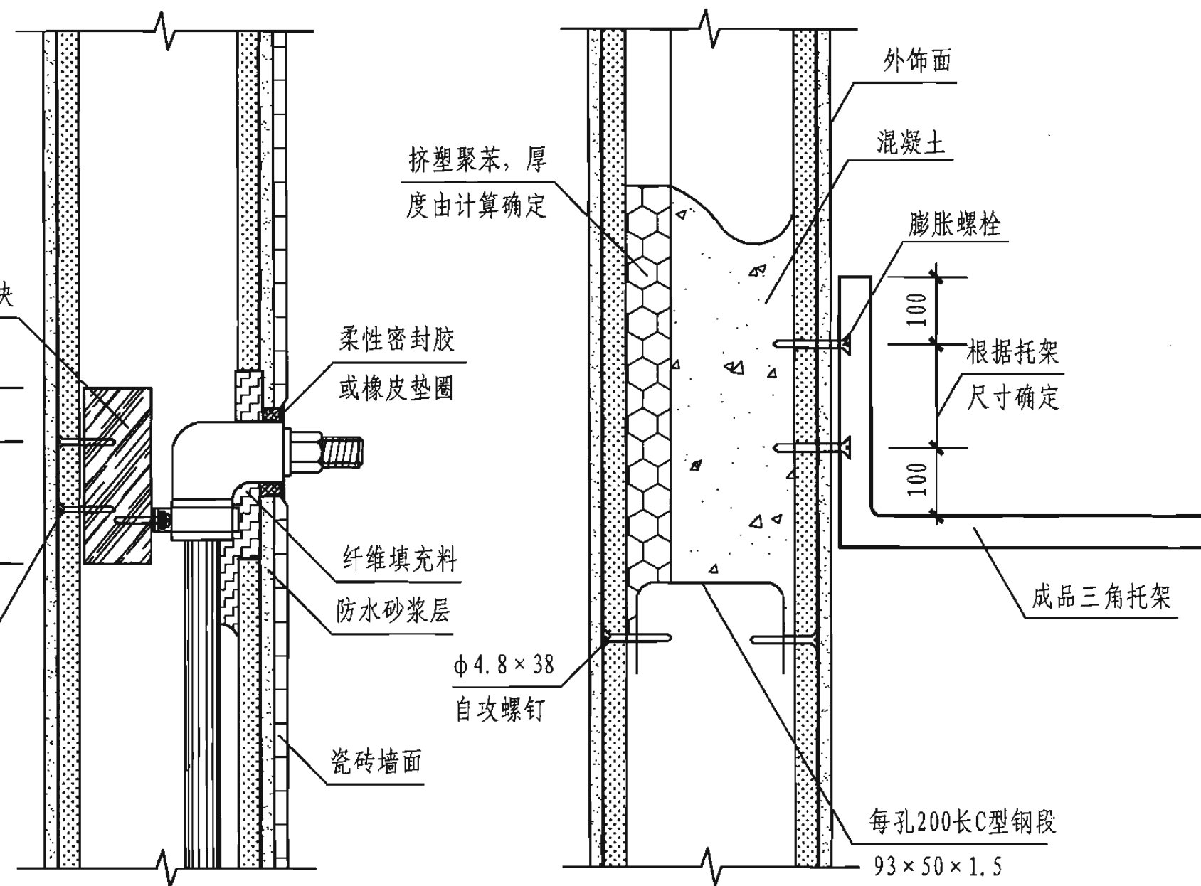
2 墙内穿管安装节点
