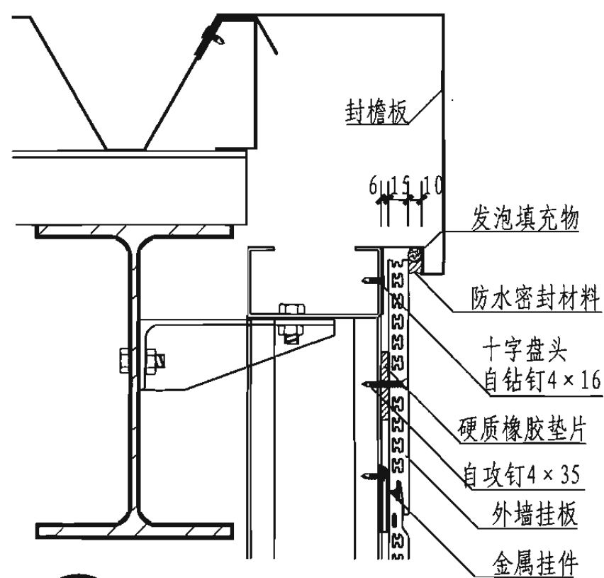
1 檐口
