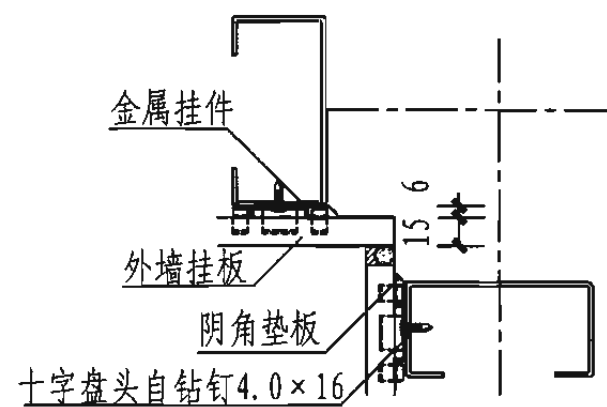
10 阴角
