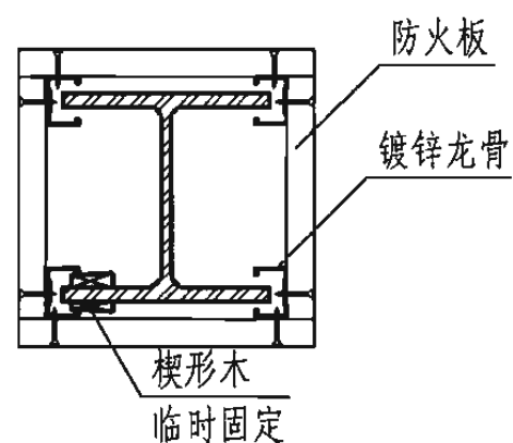
1 防火板包柱
