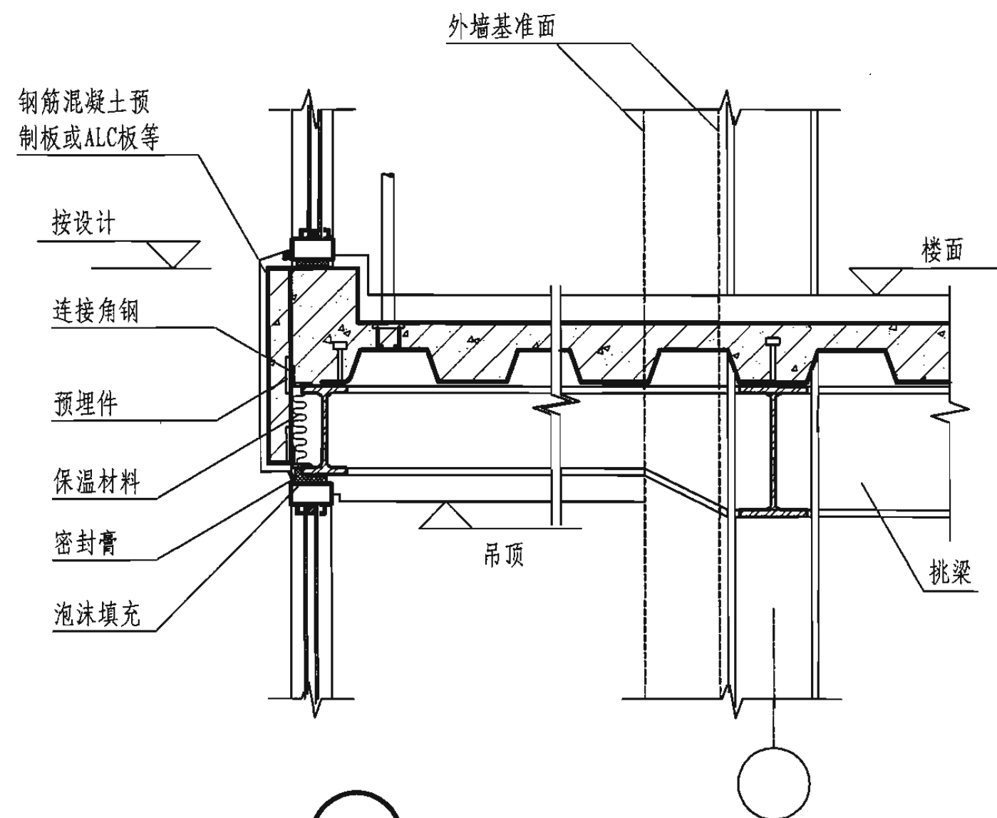
2 挑梁式封闭阳台
