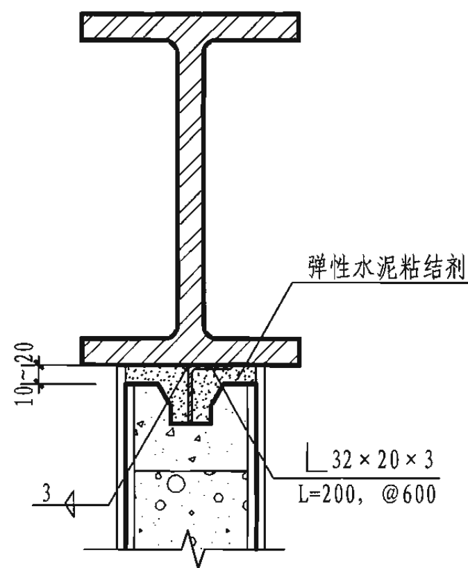
2 单板与钢梁连接 (二)
