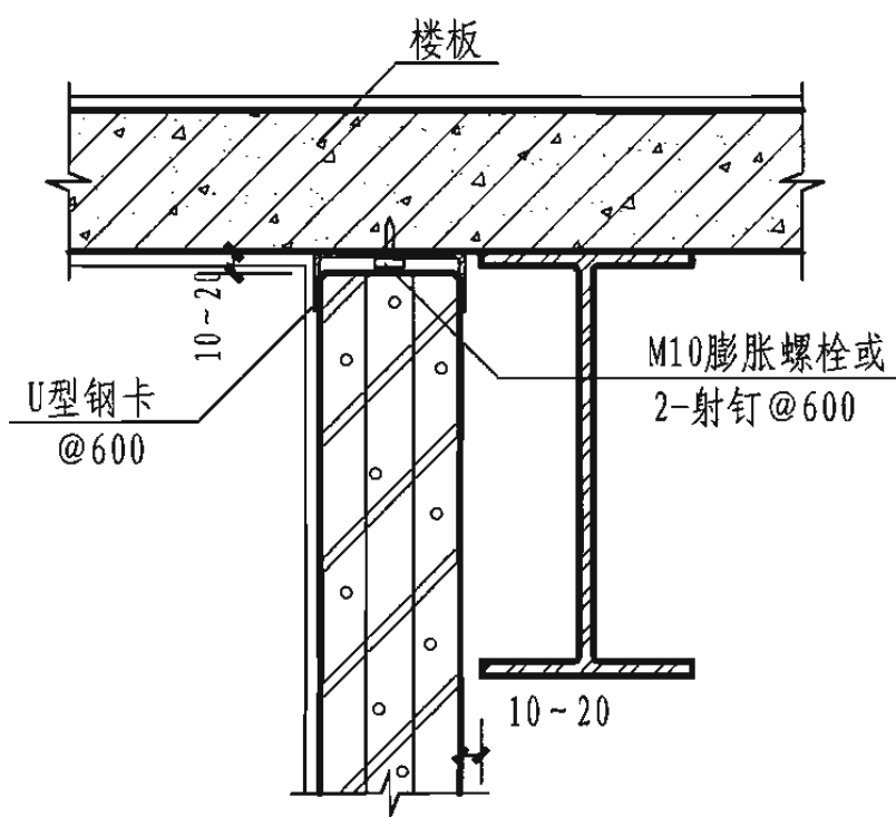
5 隔墙偏置连接
