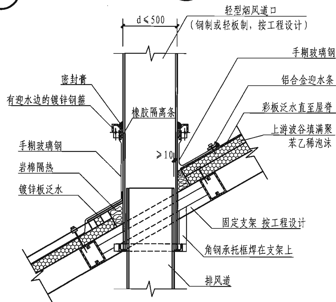
4 排风道——夹芯板屋面
