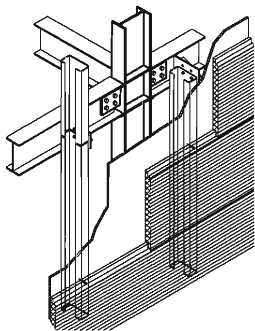
佳合金属面压花复合板安装组装图
