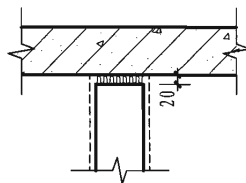
15 砌体墙与板底连接
