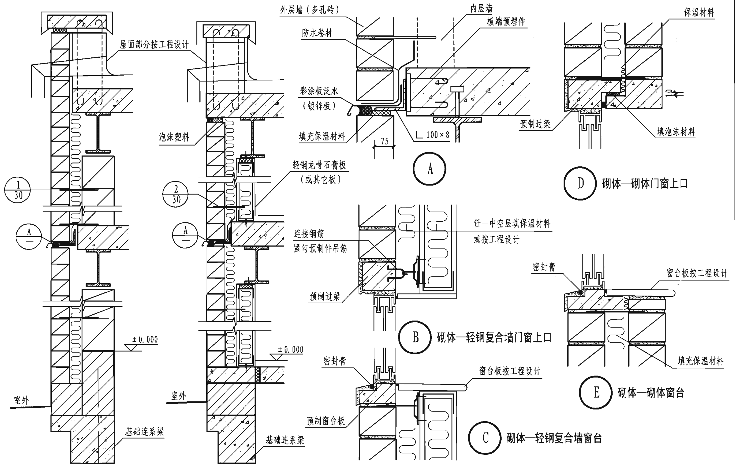
1 砌体—砌体 2 砌体—轻钢复合墙
