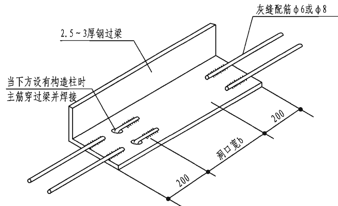
A 钢过梁与水平钢筋、构造柱的连接
