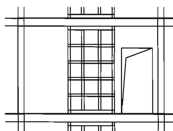
带加劲肋的钢板剪力墙 (可用于含洞口外墙)
