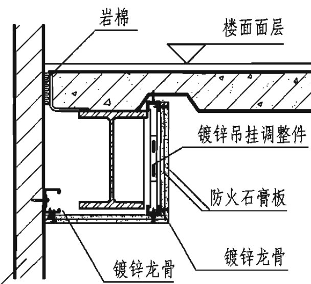
7 防火石膏板包梁
