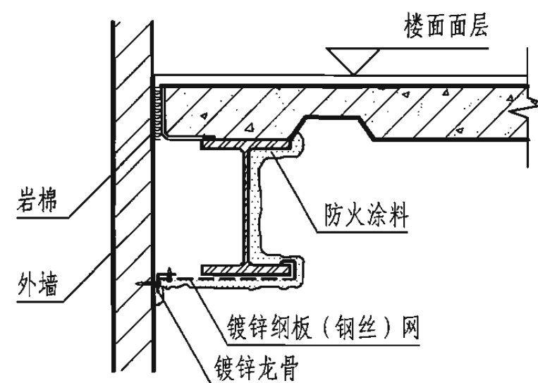
7 外沿梁防火涂料（喷涂）
