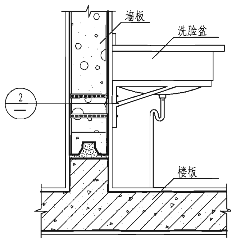
1 洗脸盆连接
