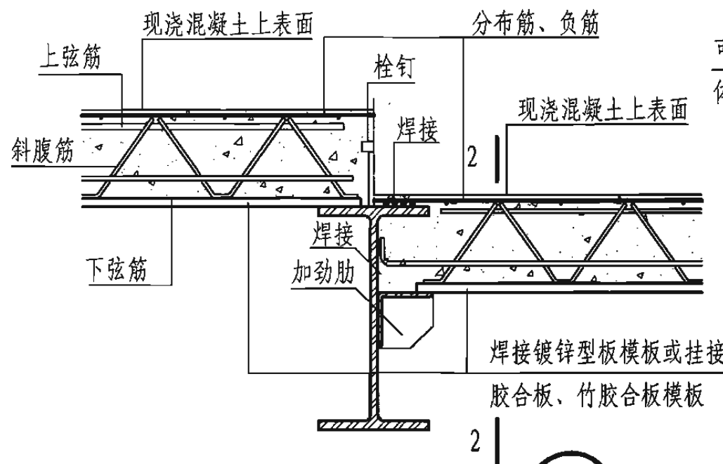
2 钢筋桁架
