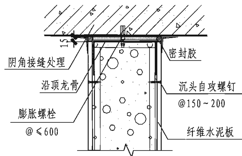
2 轻质灌浆内隔墙与楼板连接
