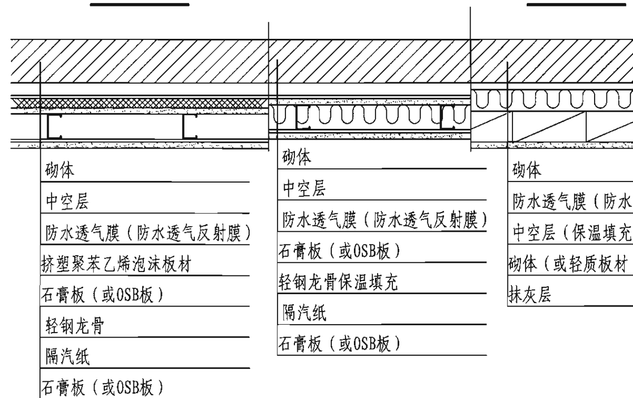
轻钢组合墙
