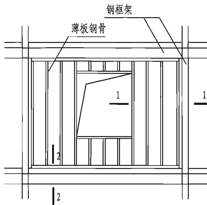
钢骨在框架中的布置
