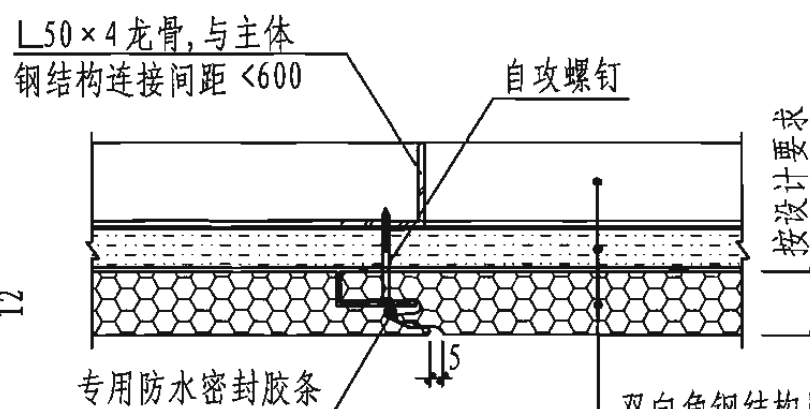
横向板缝连接
