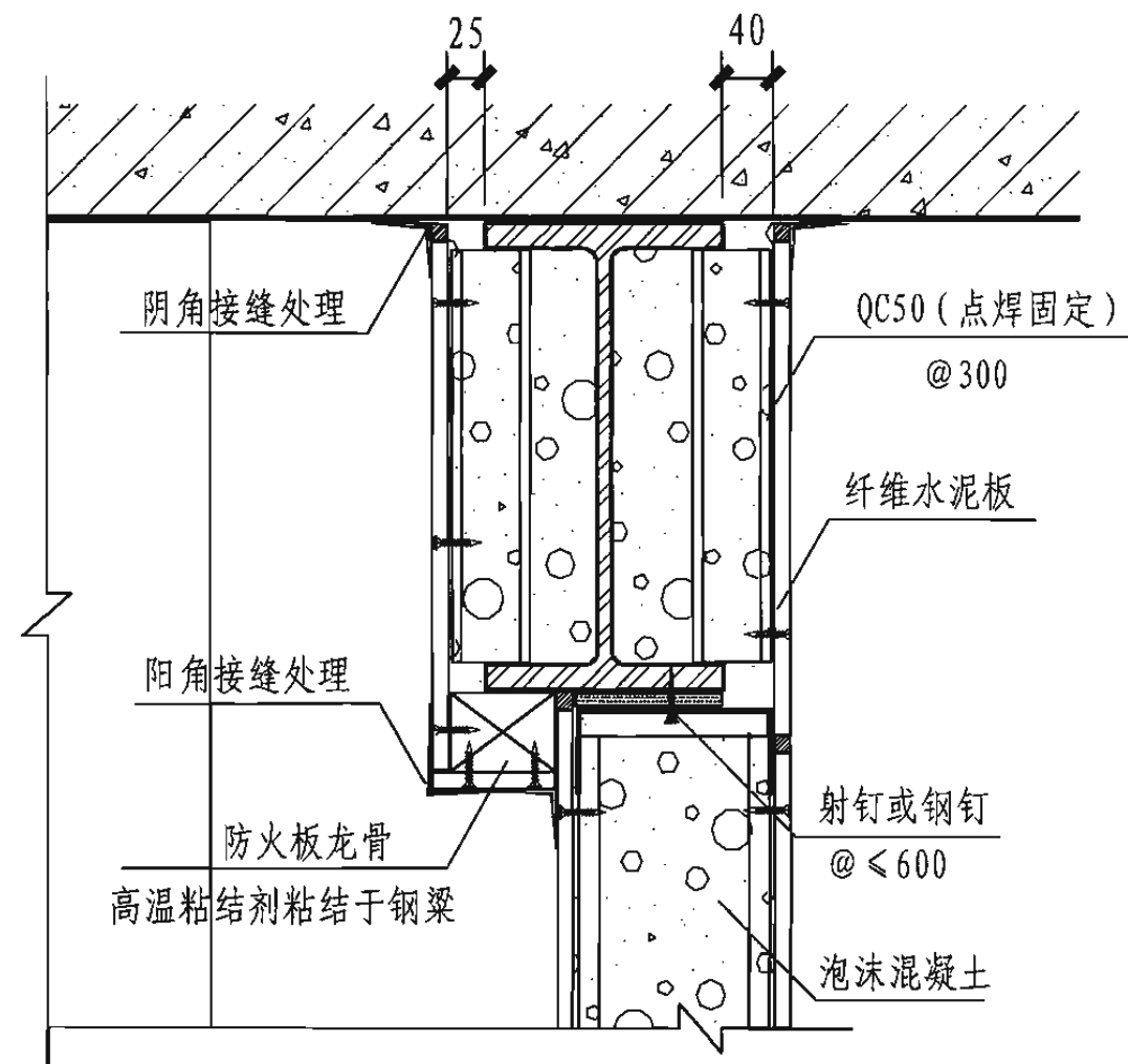
1-1
