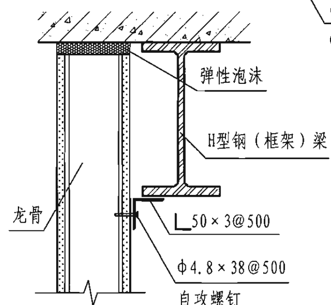
5 墙板与钢梁连接
