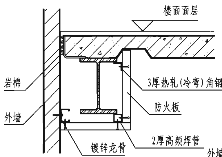
6 防火板包梁
