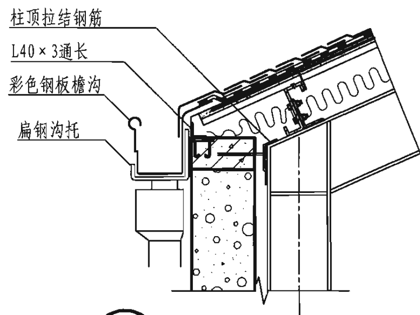
2 油毡瓦屋顶外排水檐口
