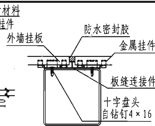
5 板缝
