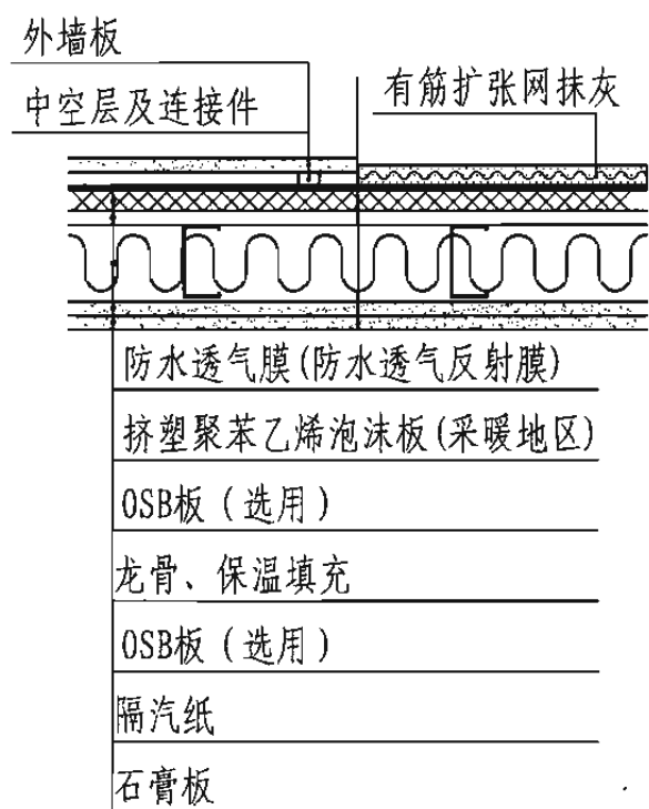
轻钢组合墙
