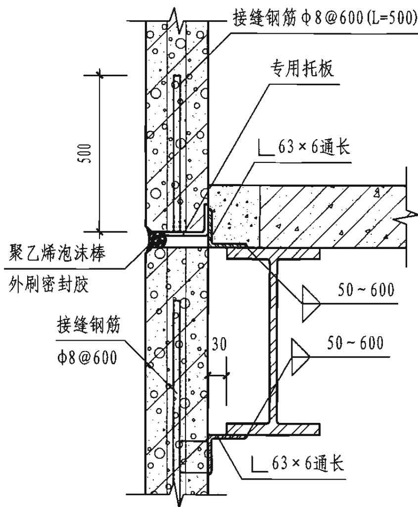
2 外墙竖板楼层部位
