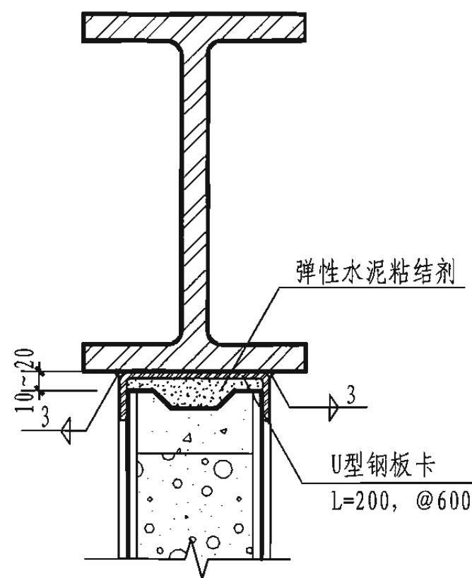
1 单板与钢梁连接 (一)
