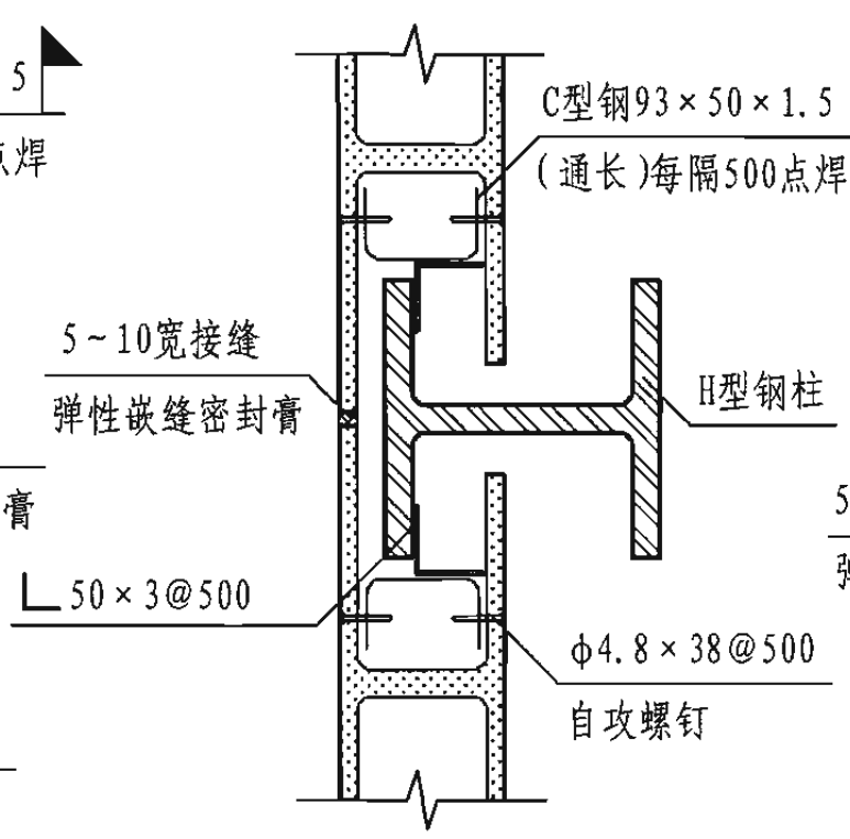
3 墙板与钢柱连接
