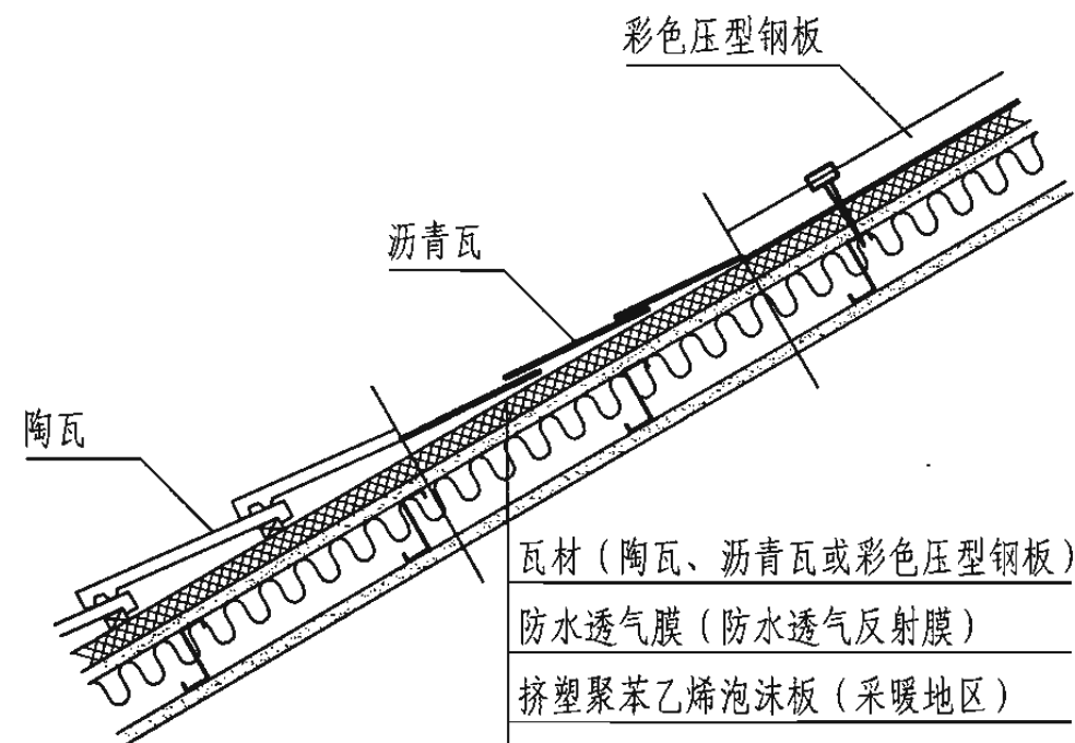
坡屋顶构造
