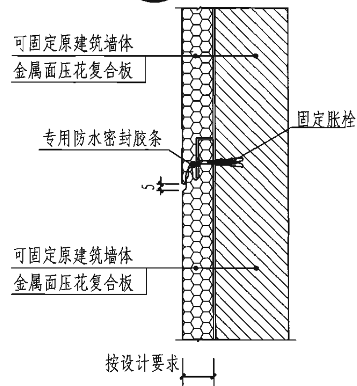
与实体墙连接
