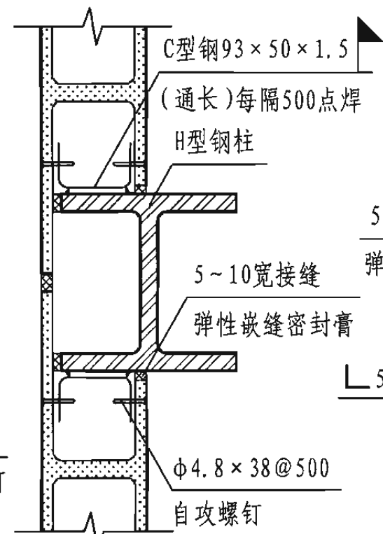
2 墙板与钢柱连接
