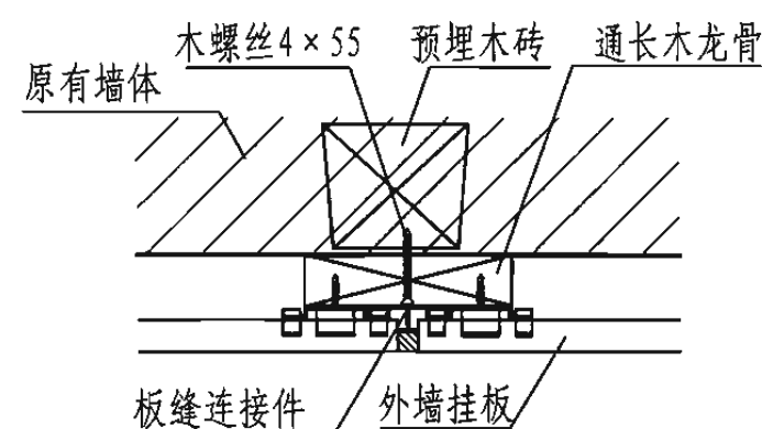
6 接缝
