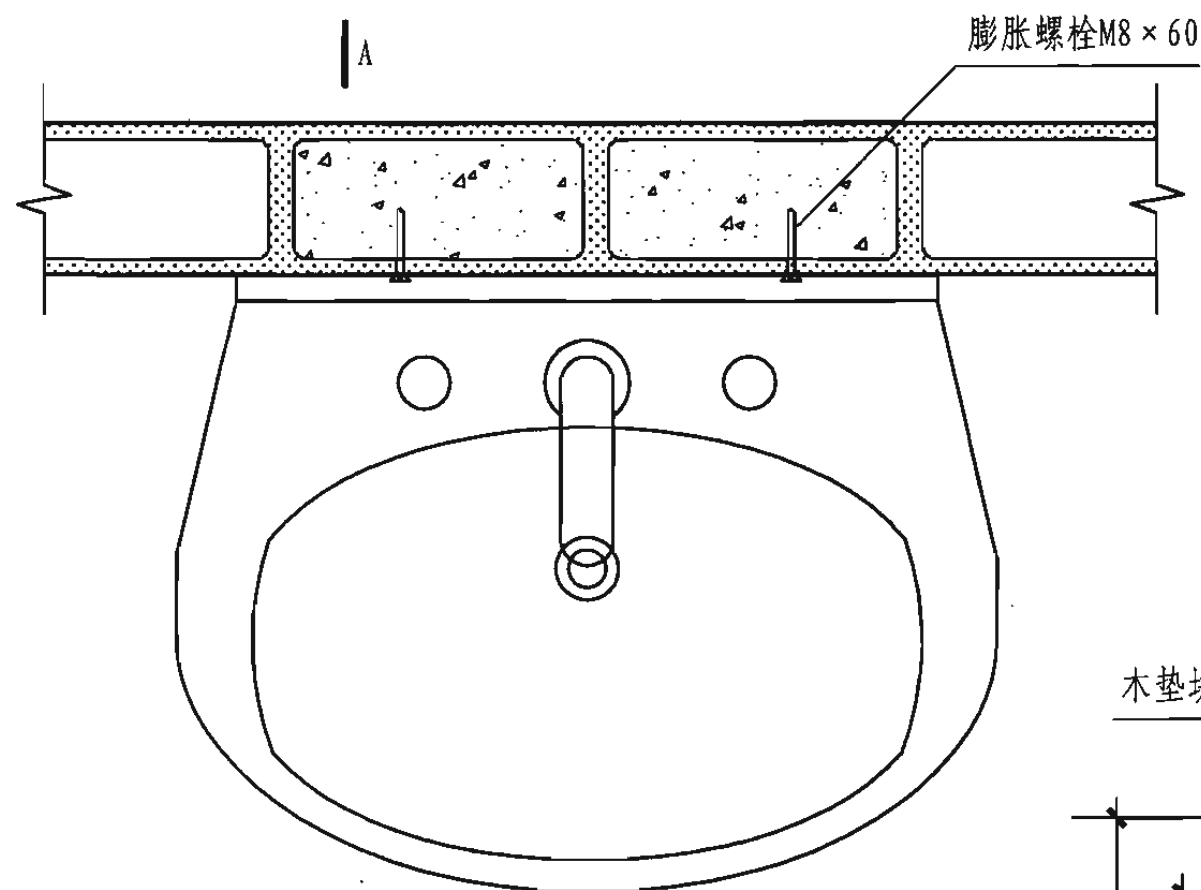
1 墙板上固定脸盆平面图
