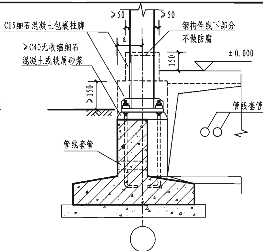
条形基础 (适用多层)
