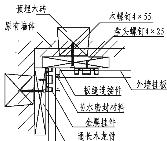
8 阴角
