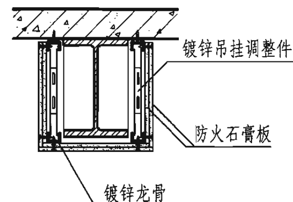
8 防火石膏板包梁
