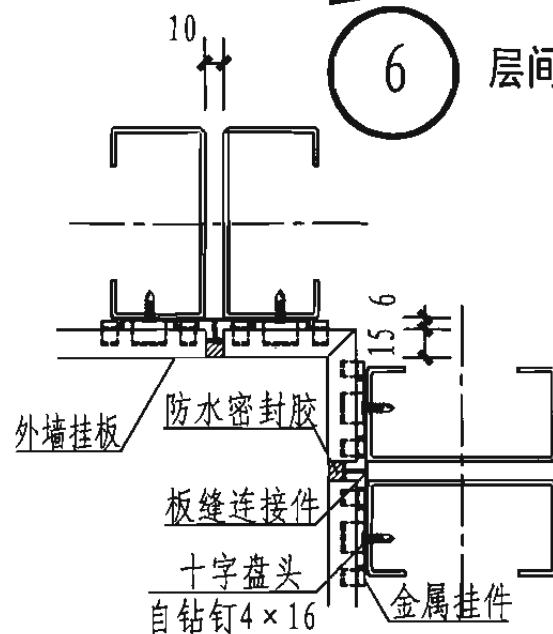
9 阴角
