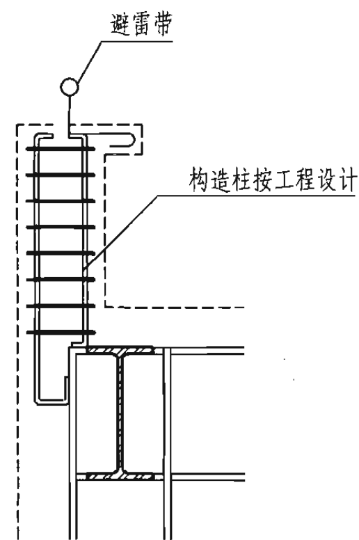
4 现浇女儿墙构造柱配筋
