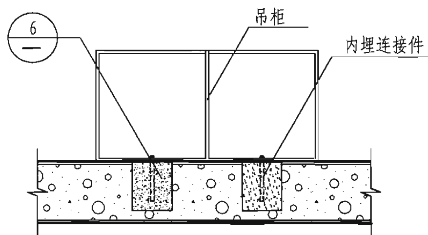
4 吊柜连接
