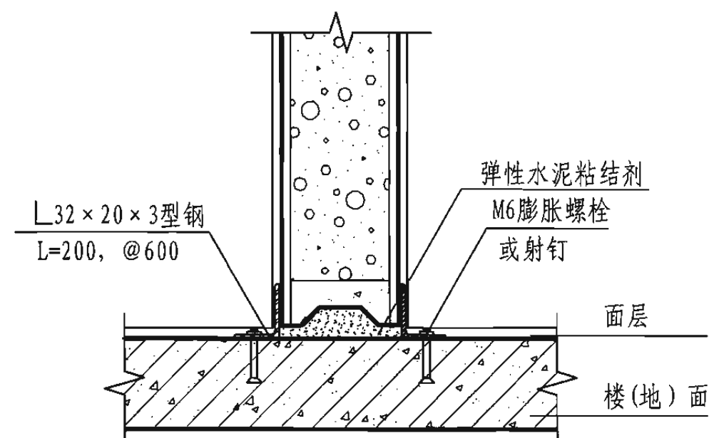
2 墙板与楼板连接(一)
