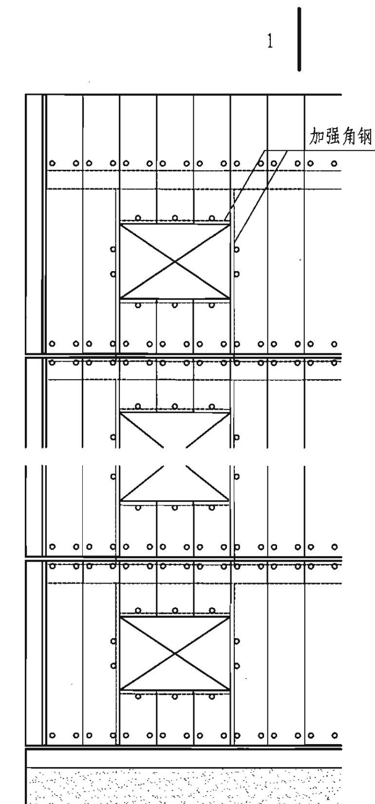
外墙立面(一)
