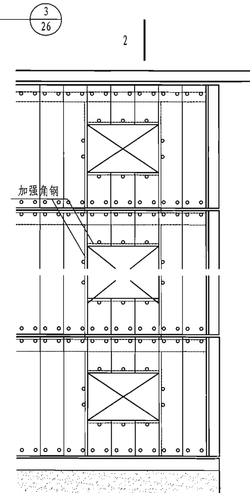
外墙立面(二)
