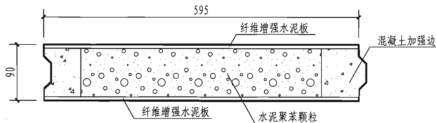
墙板构造图
