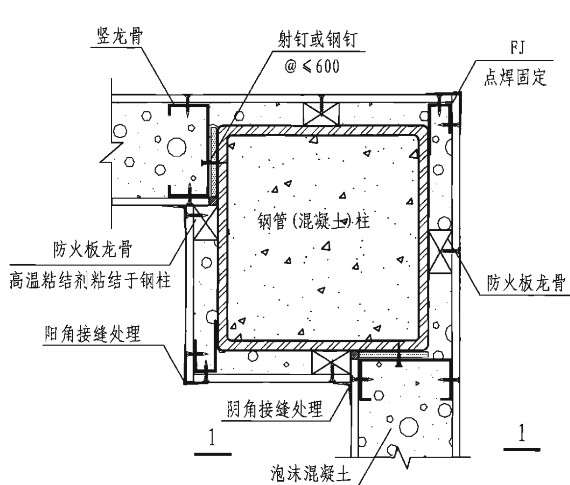
1 轻质灌浆内隔墙与钢柱连接
