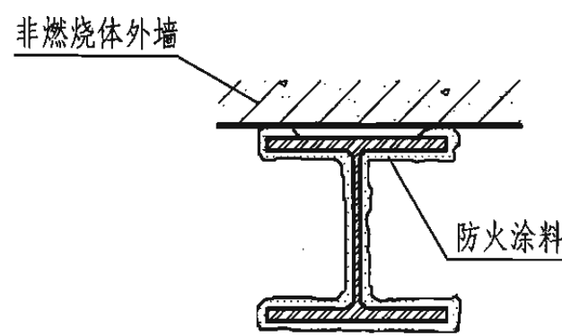
9 防火涂料包柱
