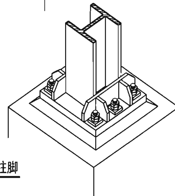
铰接柱脚
