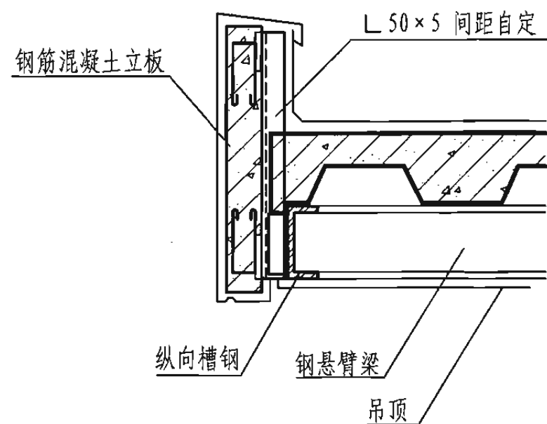
1 预制挑檐板
