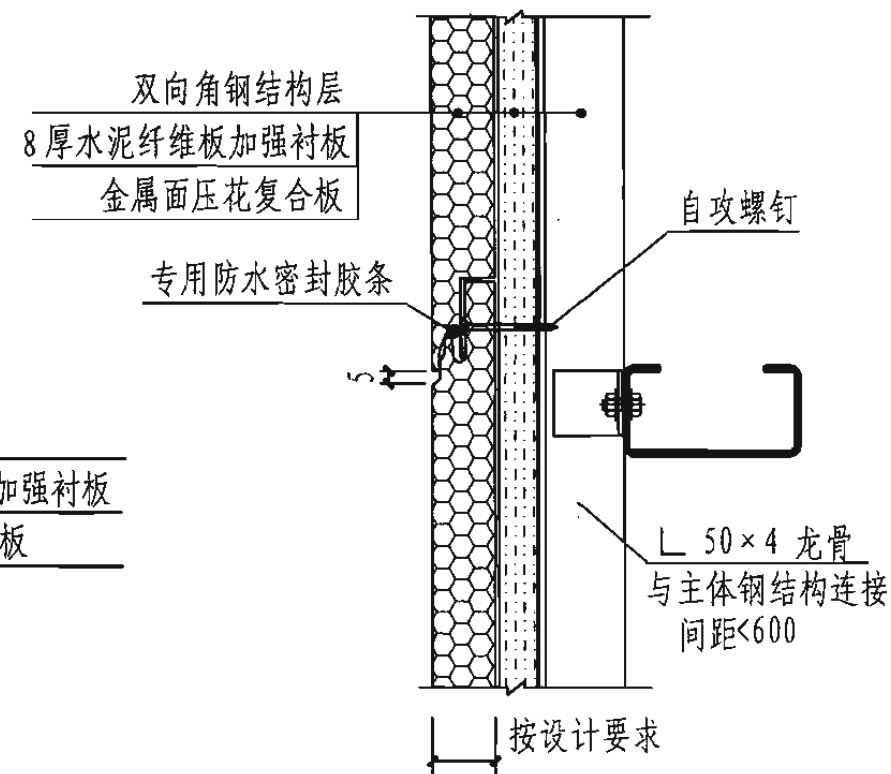
与钢骨架连接
