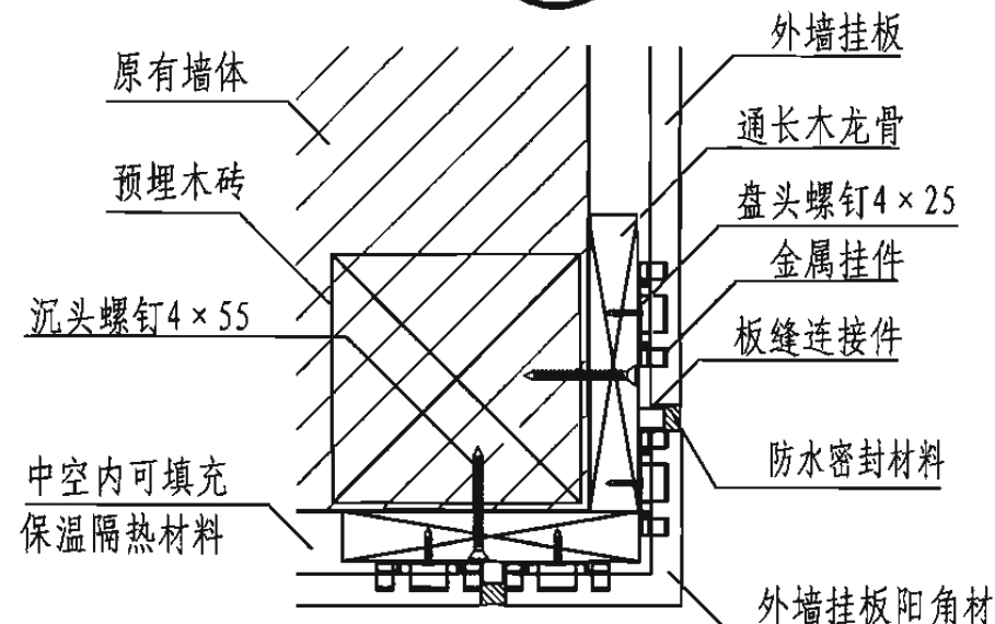
9 阳角
