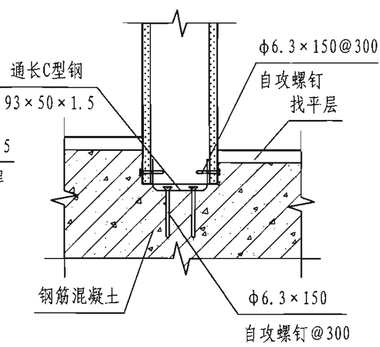
8 墙板与钢梁连接
