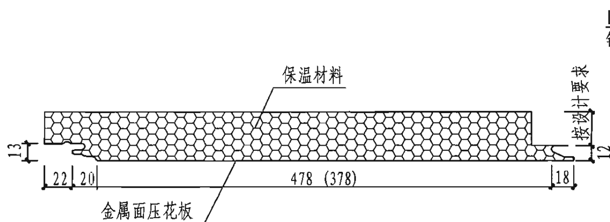
金属面压花复合板型截面图
