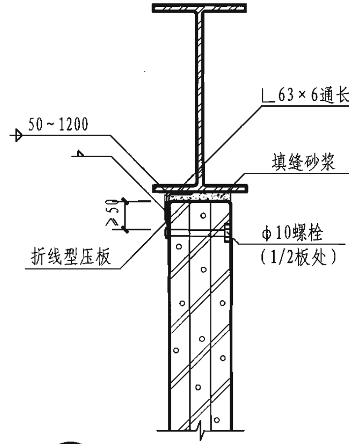
3 隔墙与钢梁对中连接
