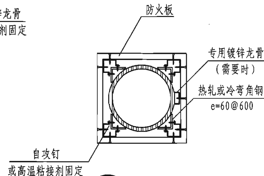
4 防火板包柱
